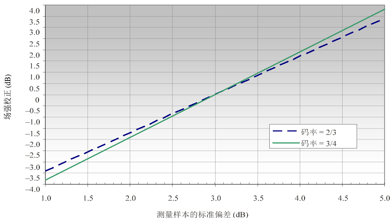
图 25 因非标准接收信道而进行的校正
