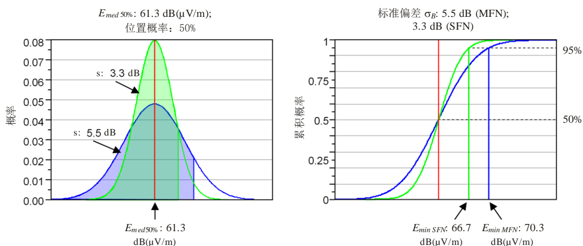
图3 网络增益
