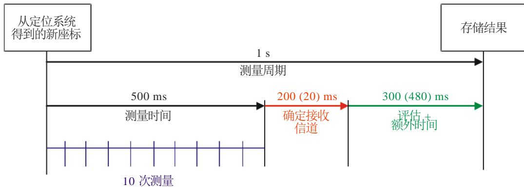
图10 单极化发射机/网络的基本时间 (便携式接收)
