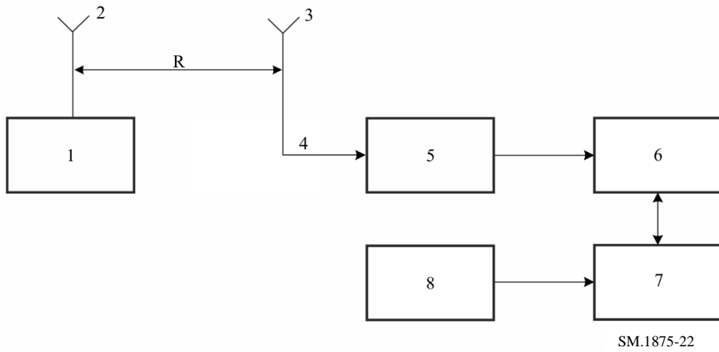
图22 设备连接图
