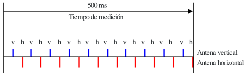
FIGURA 11 Temporización de las mediciones para SFN con polarización mixta (recepción portátil)
