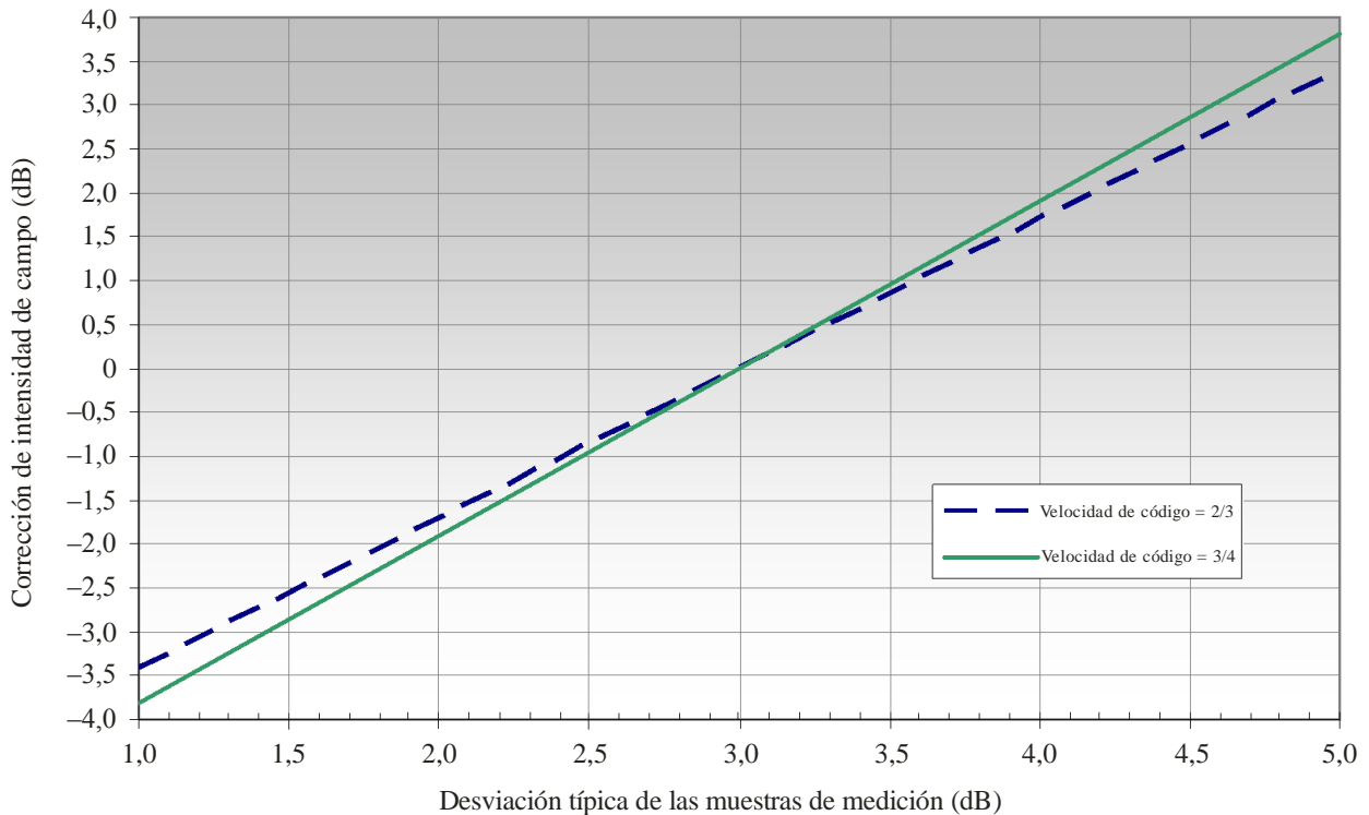
FIGURA 15 Correcciones debidas a canales de recepción no normalizados
