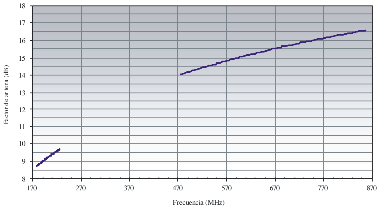
Factor de antena para la recepción de radiodifusión fija
