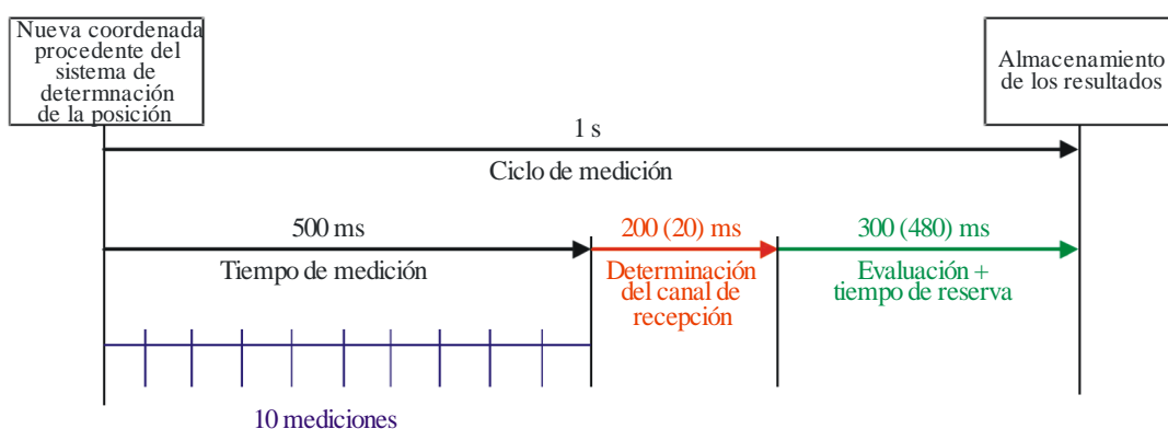
FIGURA 10 Temporización básica para los transmisores/redes con una sola polarización (recepción portátil)
