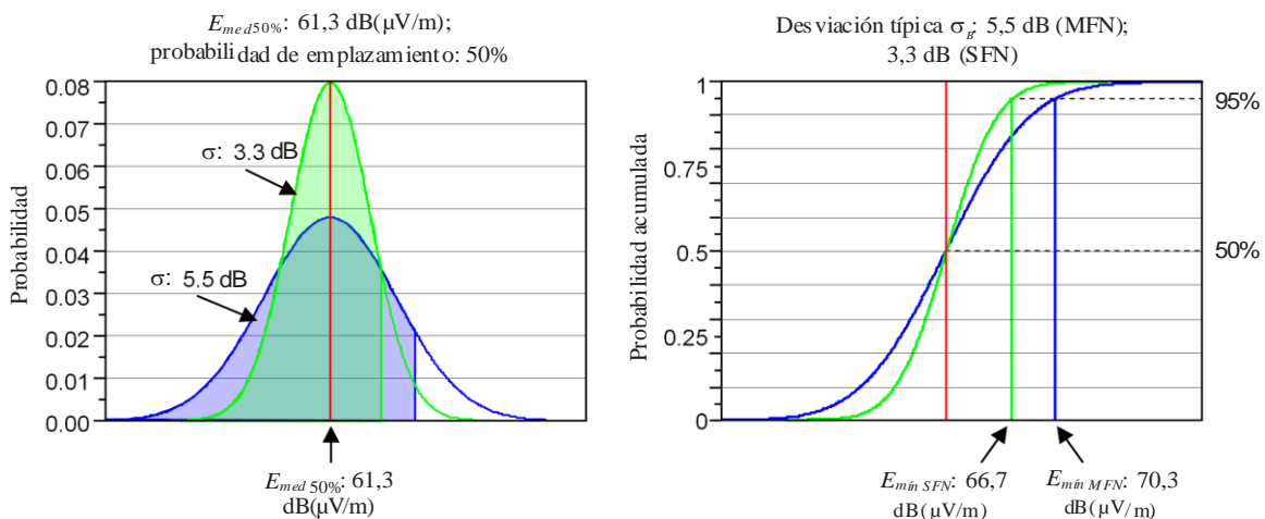
FIGURA 3 Ganancia de red
