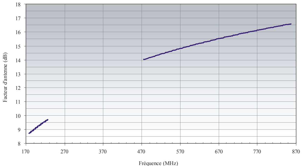
FIGURE 2 Facteur d'antenne pour la réception fixe de signaux radiodiffusés
