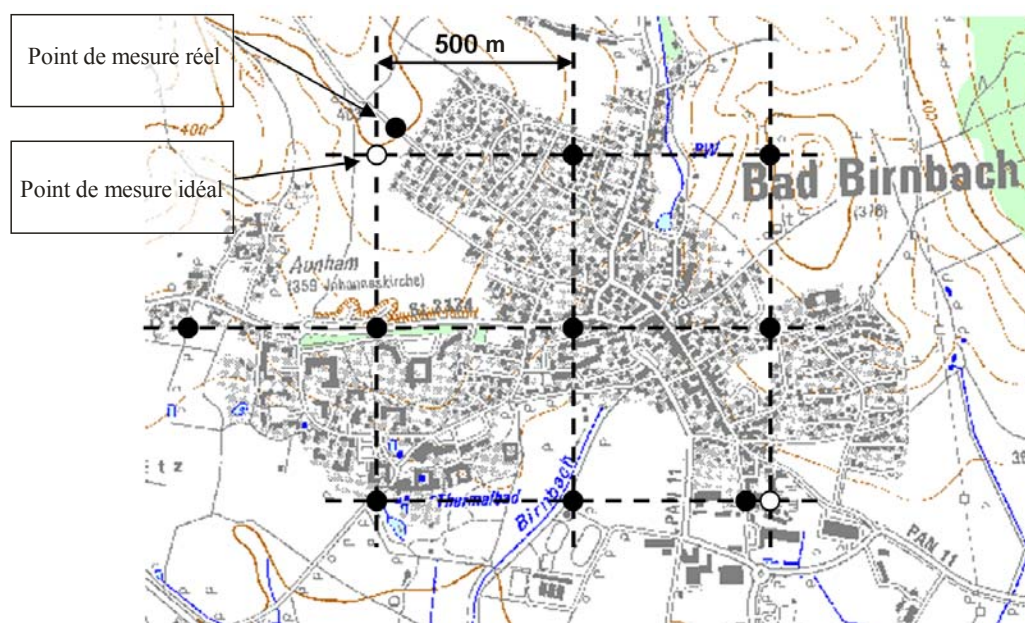
FIGURE 4 Points de mesure (réception fixe)
