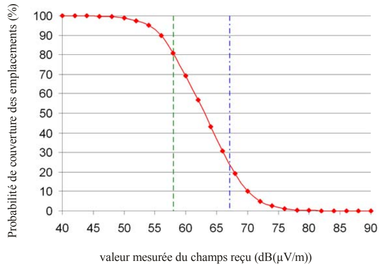
FIGURE 14 Probabilité mesurée de couverture des emplacements (réception portable)
