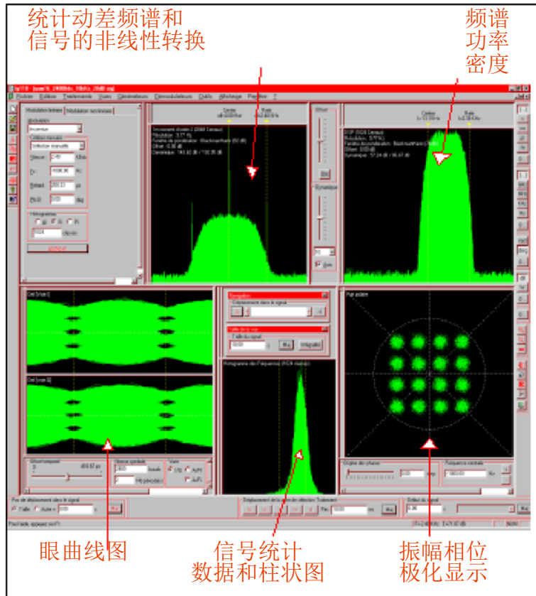
利用信号处理评估调制参数的示例
