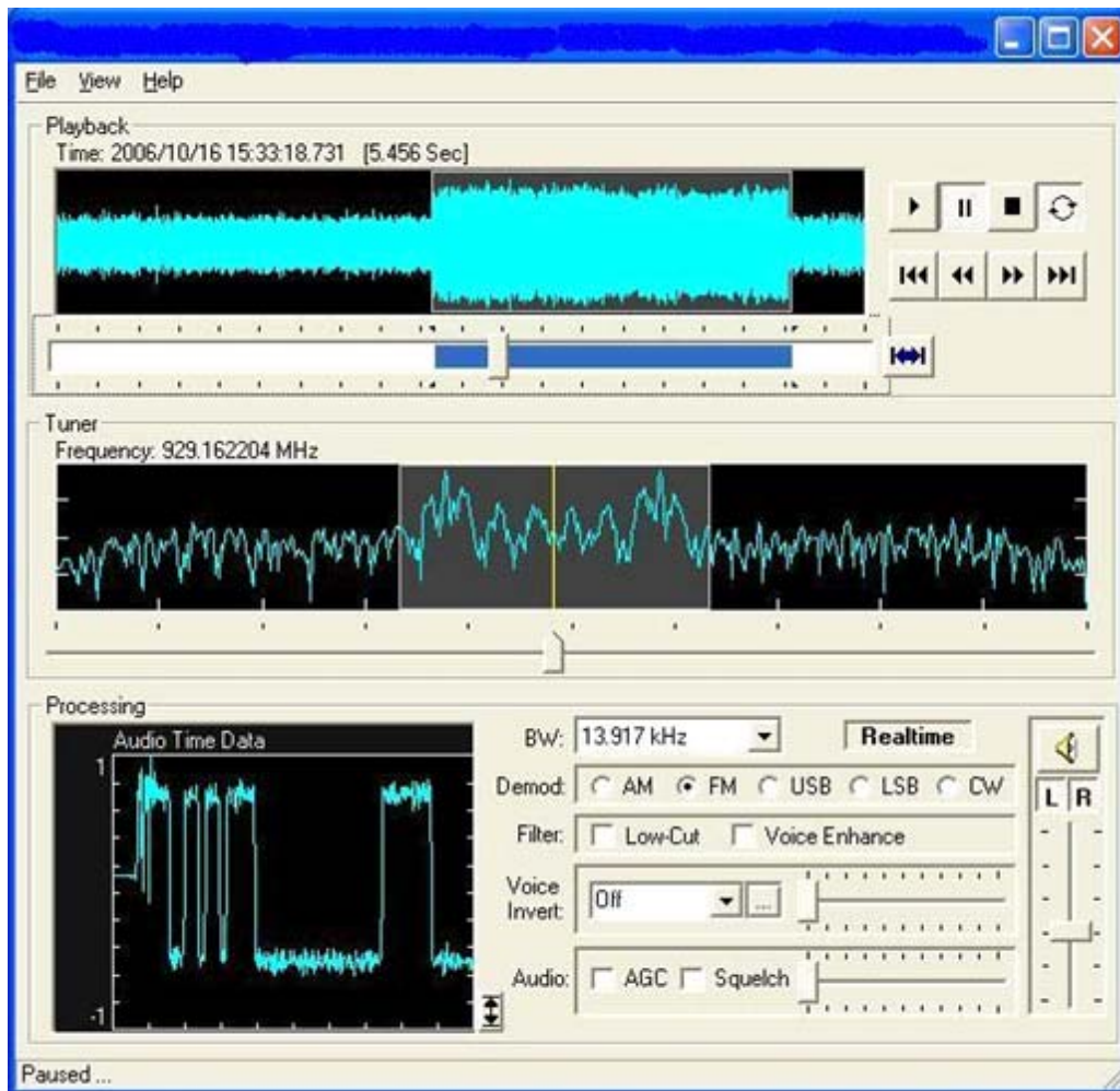
图11 I/Q音频播放器软件示例
