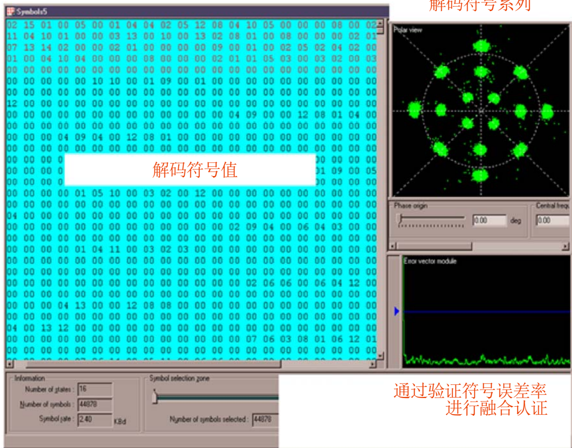
图10 解调16QAM V29信号示例
