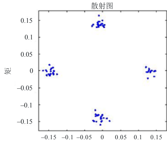
b) 主-CCPCH 信号星群
