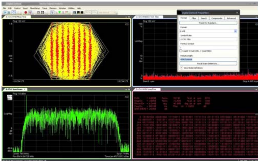
图2 说明独特频谱形状的VSA显示
