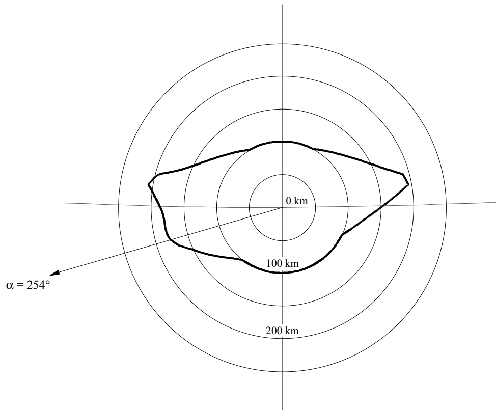
双向传播方式(1)协调区示例
