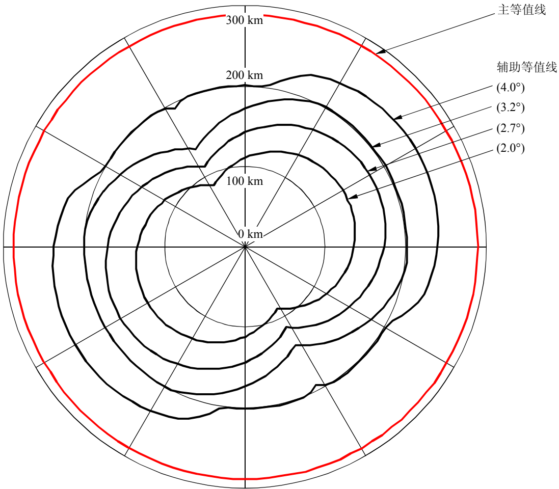
图4 传播方式(2)主等值线和辅助等值线
