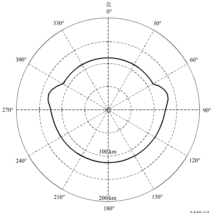
给定示例的传播方式(1)协调等值线
