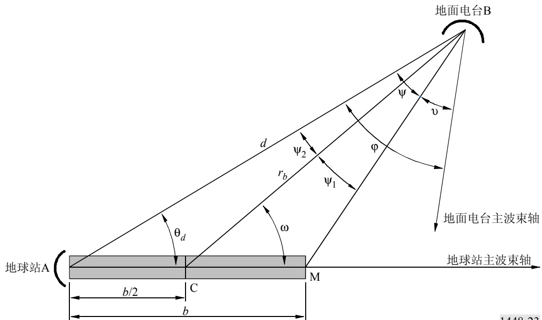
图23 水平面上的传播几何图
