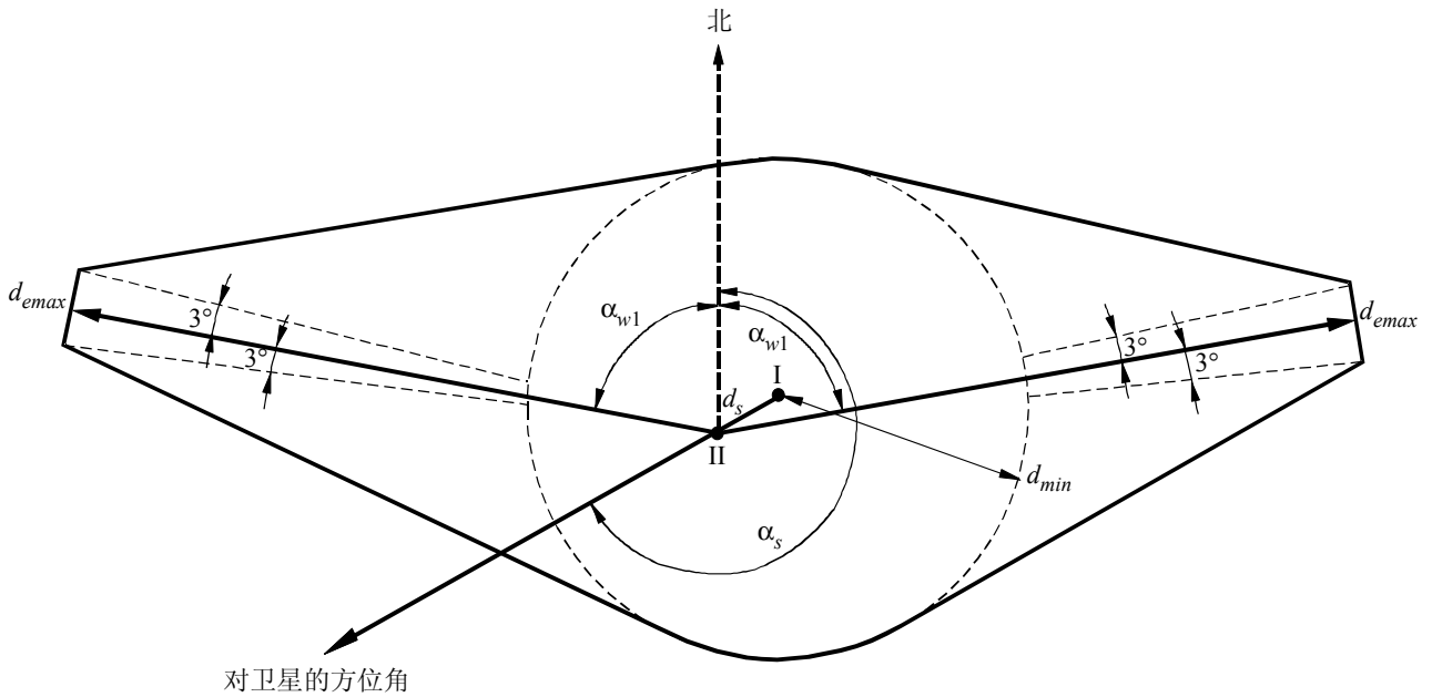
图22 双向雨散射区域示意图 (不按比例)
