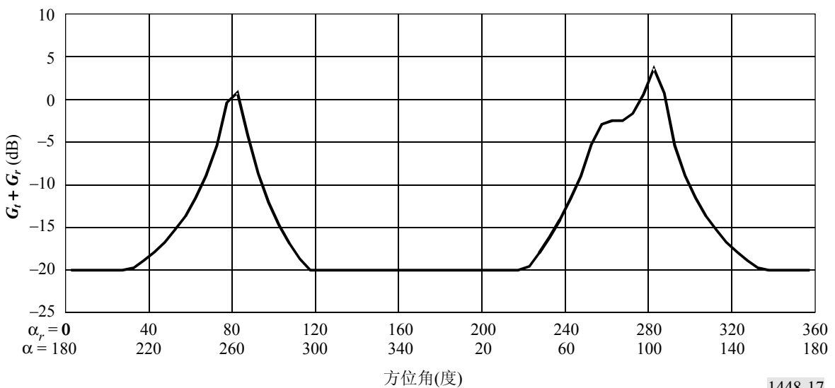
图16示例的复合水平天线增益 G_t + G_r
