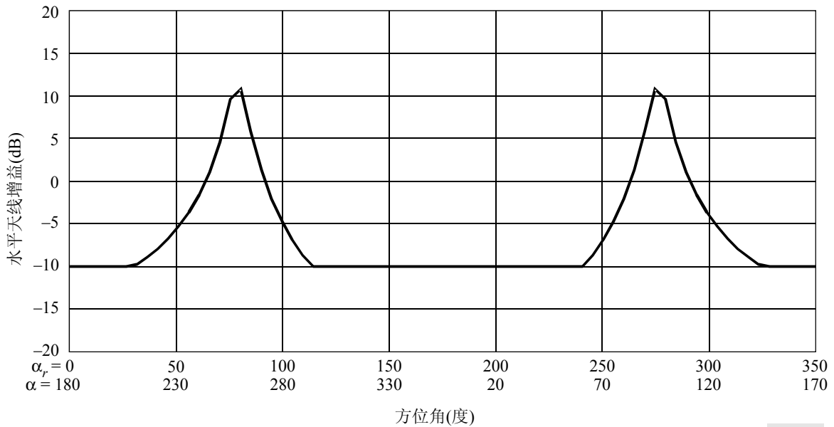
北纬40°、水平仰角0°和天线仰角最小值5°时的全弧水平天线增益示例
