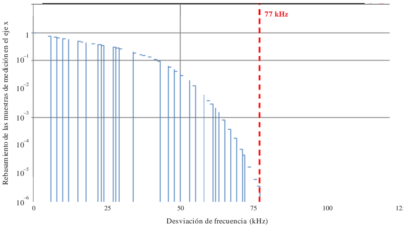
Gráfico de la distribución acumulada de la desviación (histograma), suponiendo una incertidumbre de medición de 2 kHz
