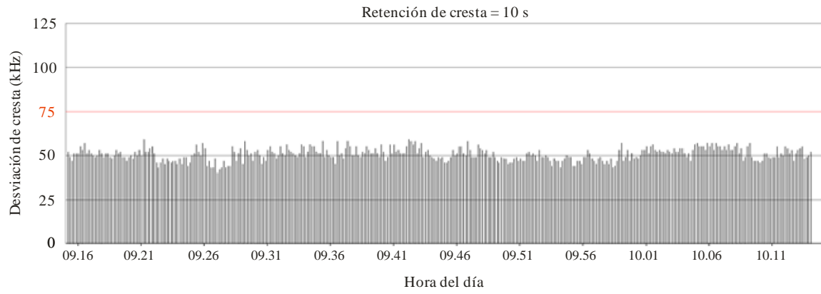
FIGURA 6 Gráfico de la desviación en función del tiempo
