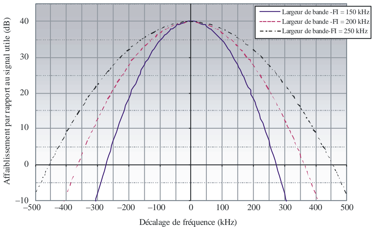
Récepteurs de mesures dotés de filtres gaussiens en fréquence FI
