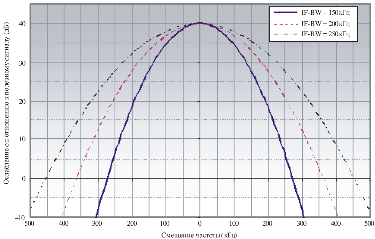
Необходимые защитные отношения для приемников с фильтрами Гаусса
