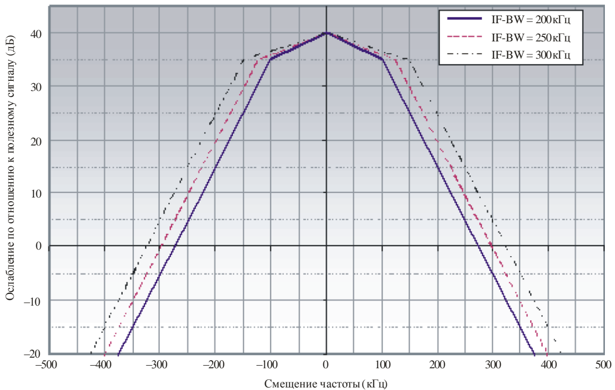
Необходимые защитные отношения для приемников с канальными фильтрами
