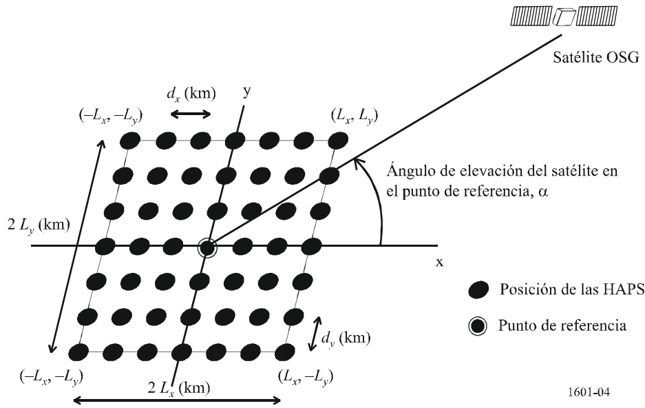
FIGURA 4 Modelo de despliegue HAPS
