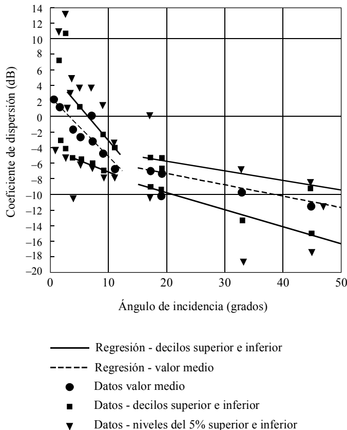
FIGURA 3 Datos del dispersímetro S-193 de Skylab
