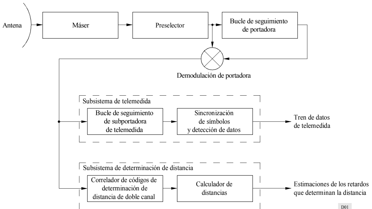
FIGURA 1 Diagrama de bloques funcional simplificado de un sistema de recepción típico de una red de espacio lejano
