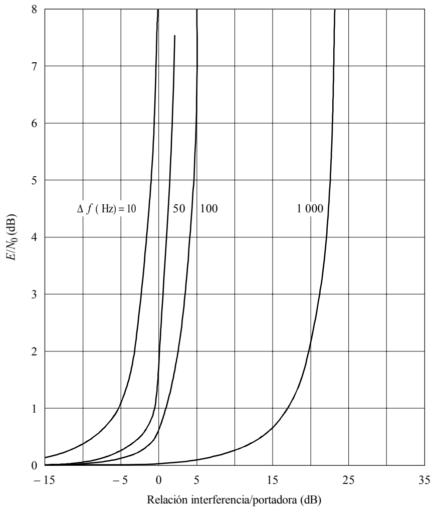
FIGURA 6 Reducción equivalente en la relación señal de determinación de distancia/ruido, E/N_0 , por efecto de error de fase y temblor de fase en el bucle de portadora, en función de la relación interferencia/portadora para diferentes valores del desplazamiento de frecuencia
