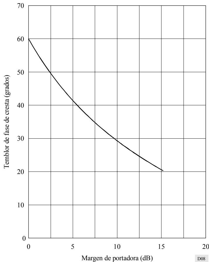
Temblo de fase de cresta en función del margen de portadora
