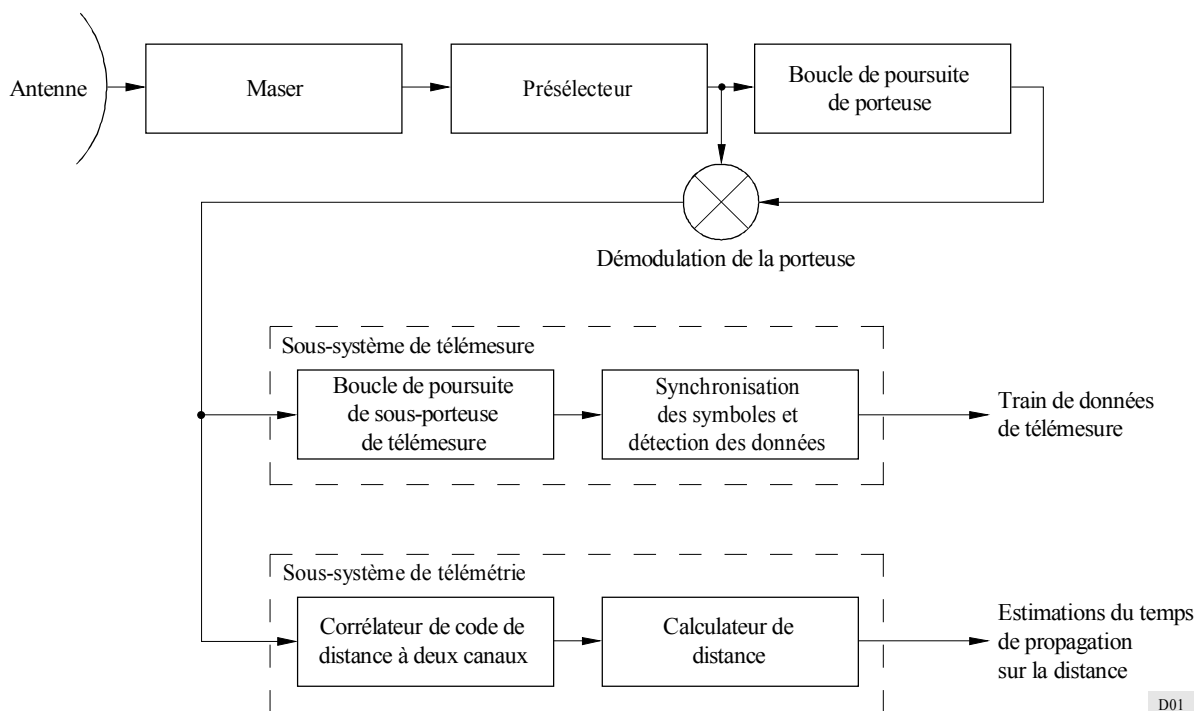
Schéma de principe fonctionnel simplifié pour un système de réception type du réseau d'espace lointain
