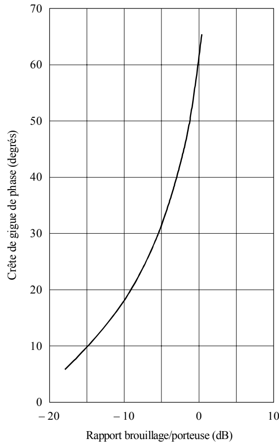
FIGURE 3 Crête de gigue de phase en fonction du rapport brouillage/porteuse
