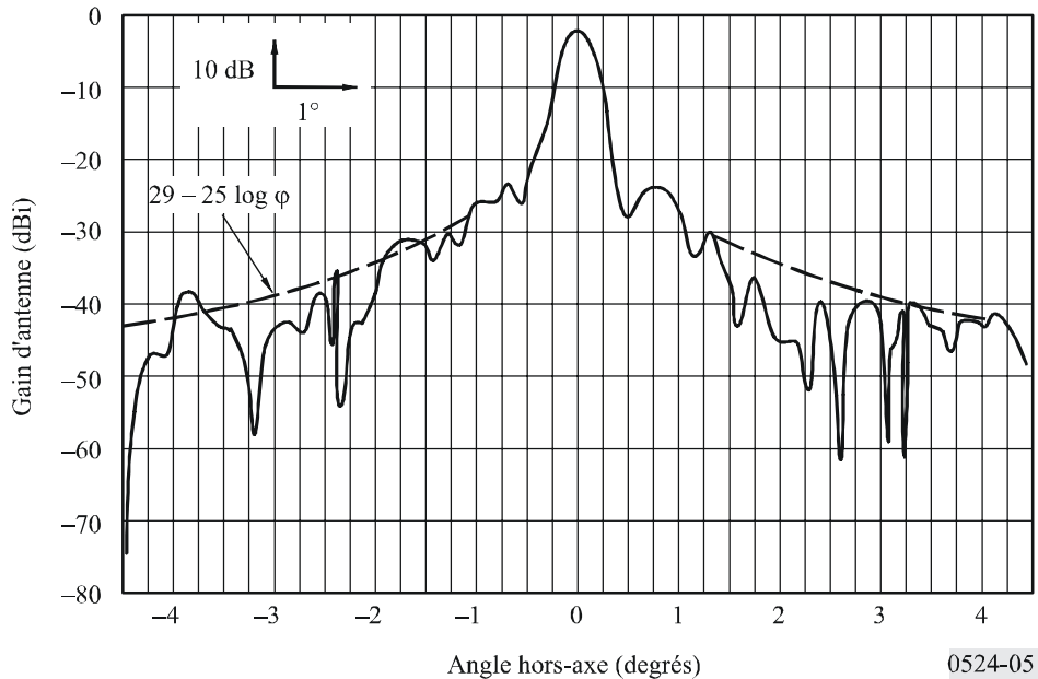
Exemple de diagramme de rayonnement d'antenne mesuré
