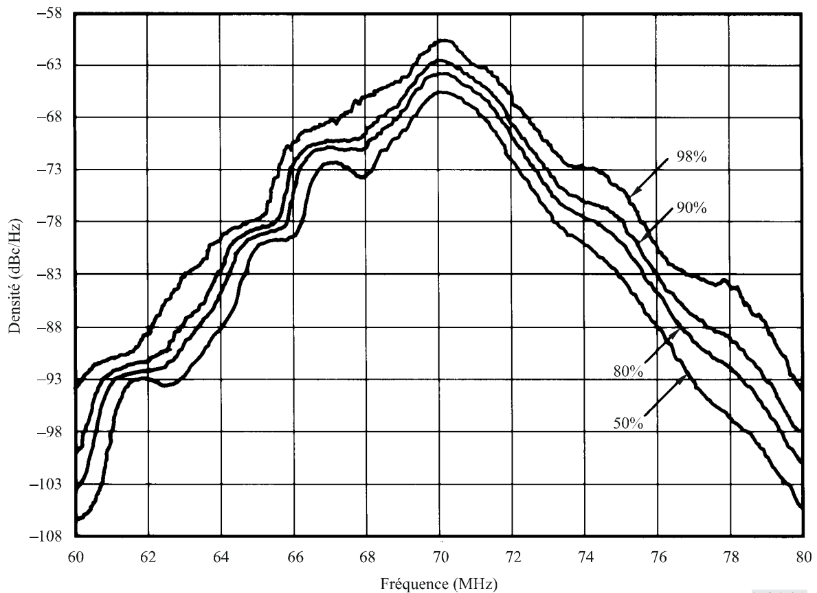
FIGURE 1 Distribution spectrale d'une porteuse TV-MF à 20 MHz modulée par un signal vidéo NTSC de programme en direct associée à une dispersion d'énergie de 1 MHz
