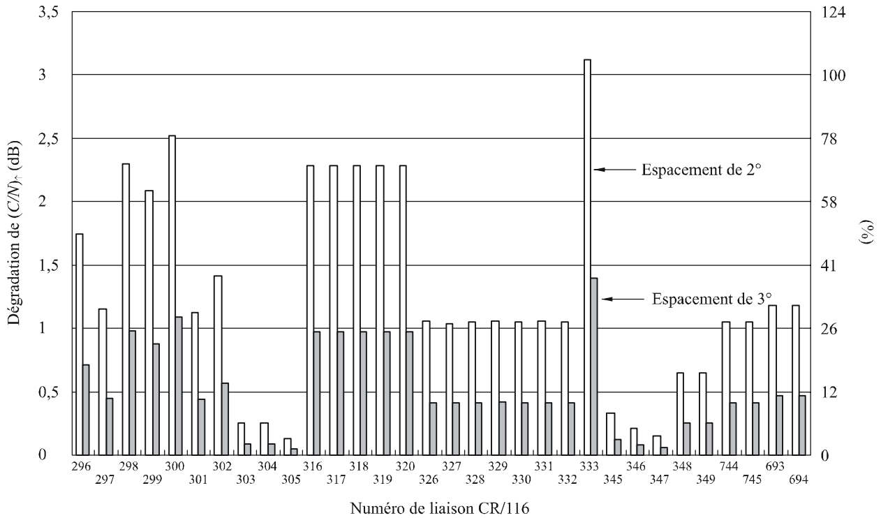
FIGURE 4 Dégradation maximale de (C/N)_f pour des liaisons CR/116 dans la bande 29,5-30 GHz, découlant d'un brouillage dû à une seule source correspondant à la limite de p.i.r.e. hors axe
