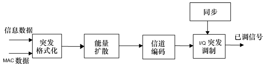
RCST 反向链路基带信号处理的方框图
