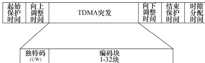
上行链路时隙和突发结构 (不按规定比例)
