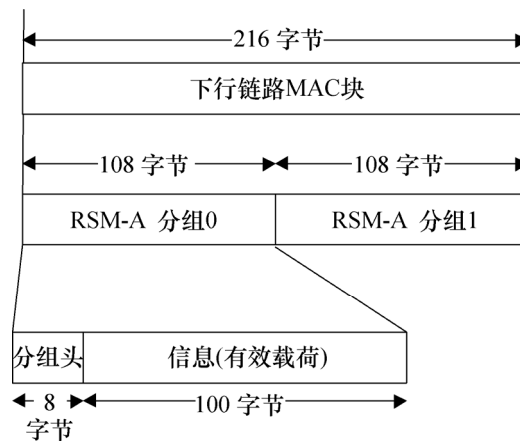
图 28 下行链路 MAC 块的组装
