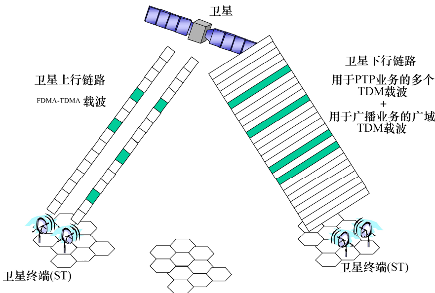
物理层概况
