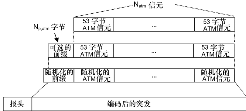
ATM TRF 突发的组成
