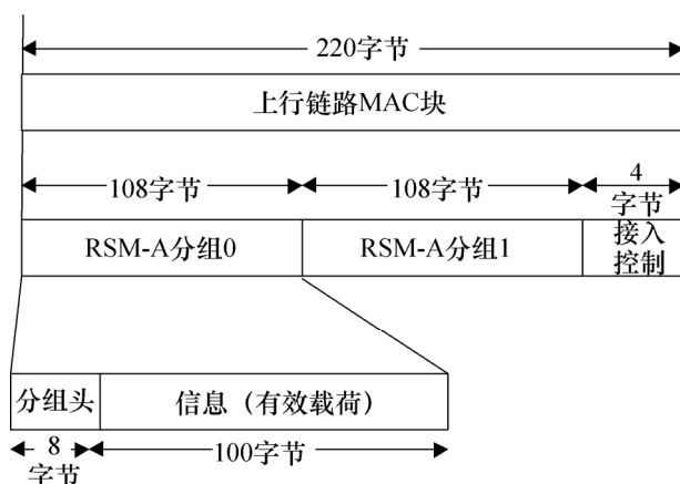
图 23 上行链路 MAC 块的组装
