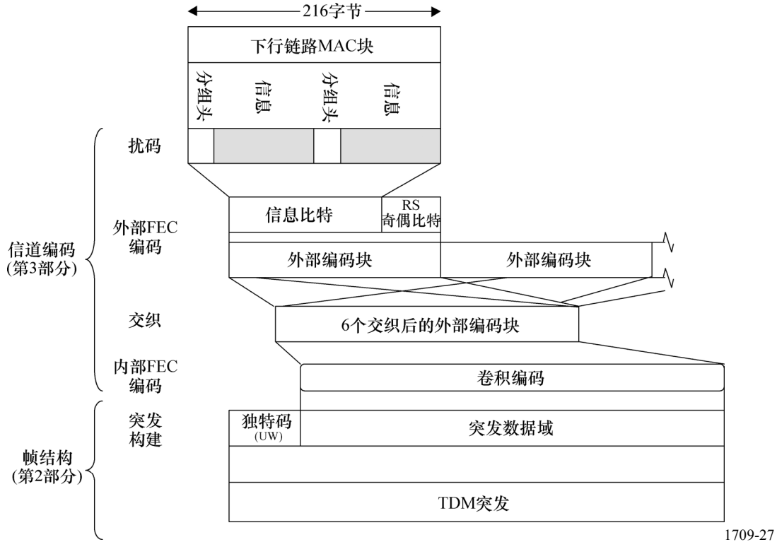
图 27 下行链路数据结构
