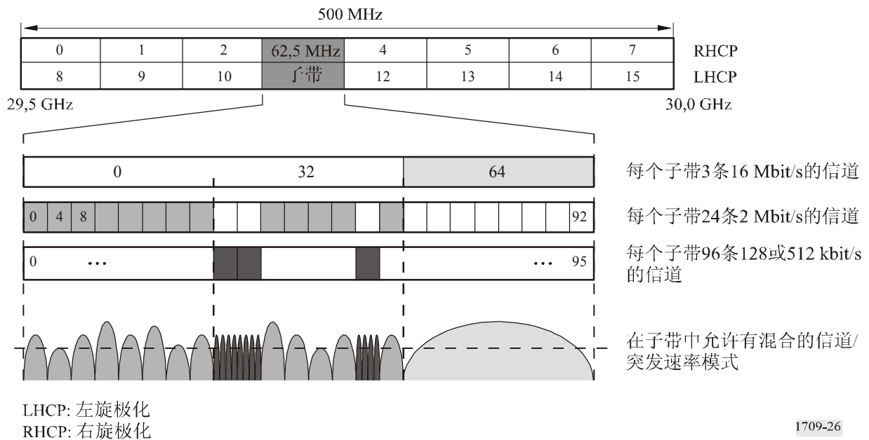
图 26 一个子带宽内上行链路载波的可能安排
