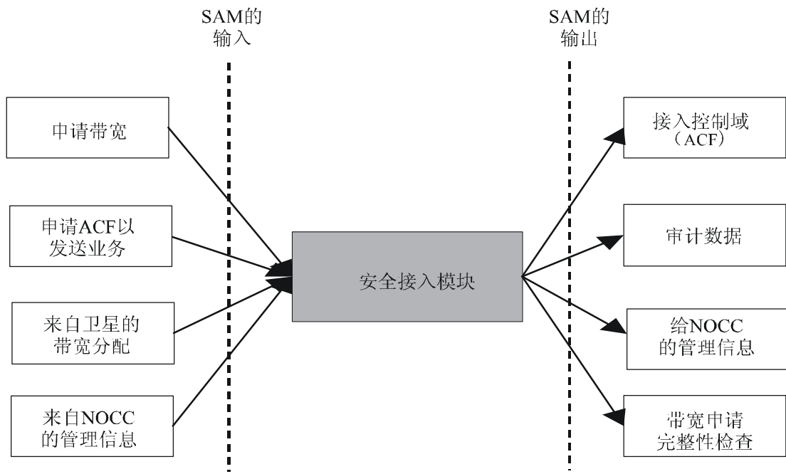
图 31 SAM 和 ST 之间的安全功能交互
