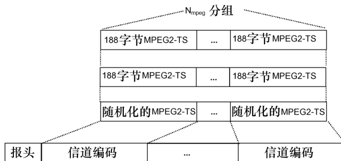
可选的携带 MPEG2-TS 分组的 TRF 突发的组成
