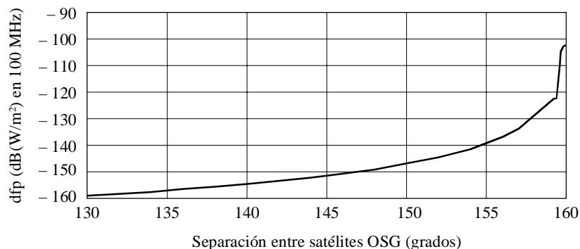
FIGURA 3 Separación entre satélites OSG admitida en función de la variación de los umbrales de dfp
