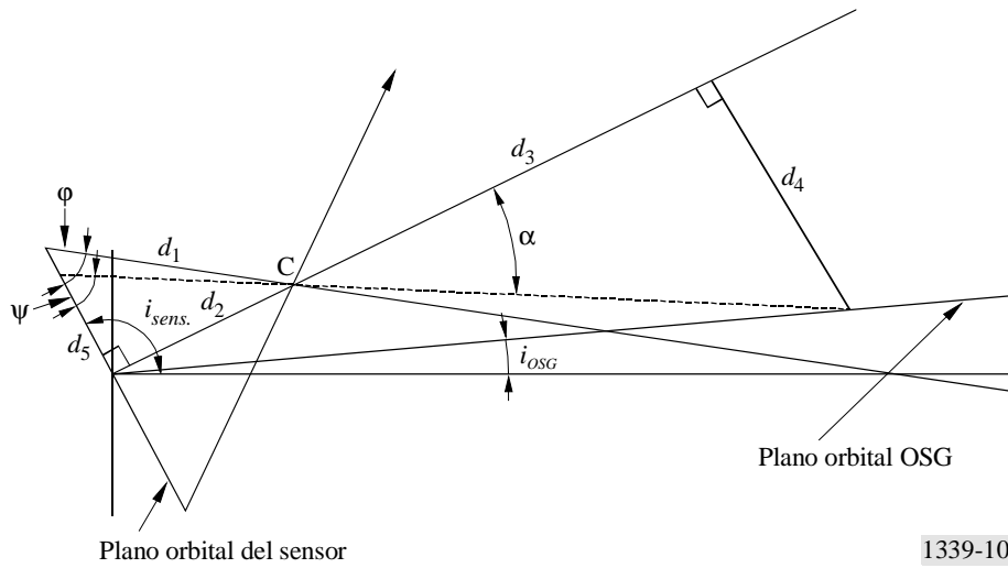
FIGURA 10 Geometría de cálculo de la latitud del sensor
