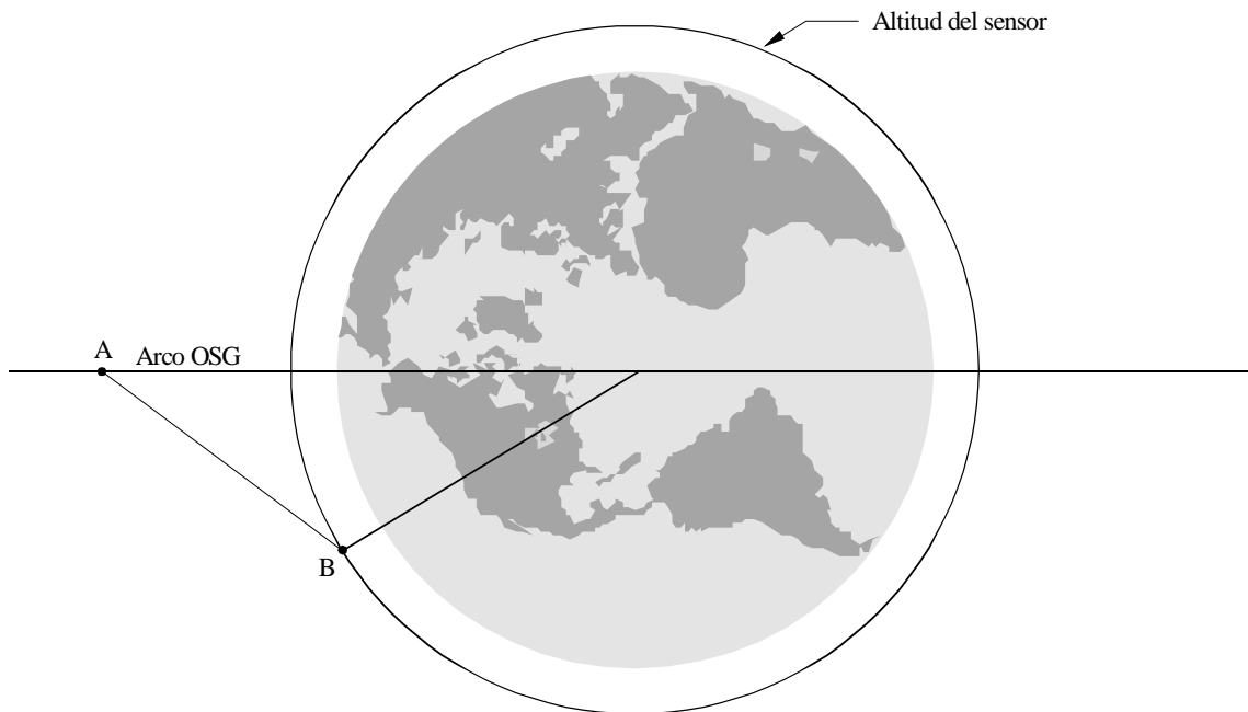
FIGURA 6 Ángulo con respecto al eje de puntería entre la OSG y el sensor pasivo Vista desde la OSG
