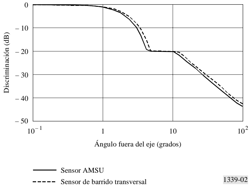
FIGURA 2 Diagramas de la antena de calibración del sensor
