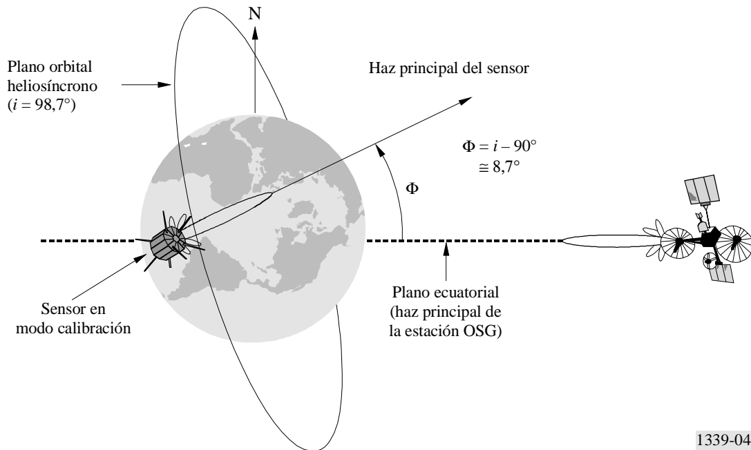
FIGURA 4 Sensor pasivo en el plano ecuatorial
