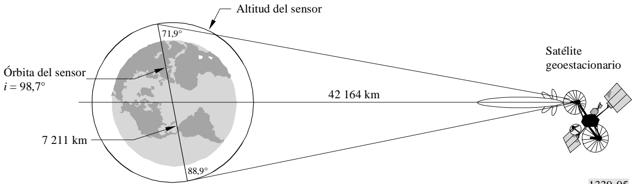
FIGURA 5 Geometría del caso 2 Vista del plano ecuatorial
