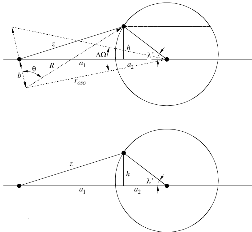
FIGURA 9 Vista a lo largo del plano OSG para la distancia a_1
