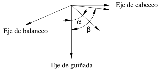
FIGURA 1 Plano de exploración del sensor pasivo
