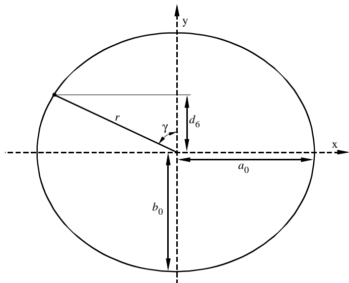
FIGURA 11 Ángulo de latitud del sensor
