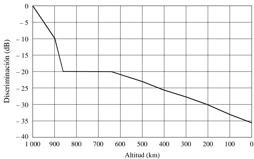
FIGURA 12 Discriminación de un sistema del SES OSG típico desde el punto 1 000 km (dfp máxima a 1 000 km)
