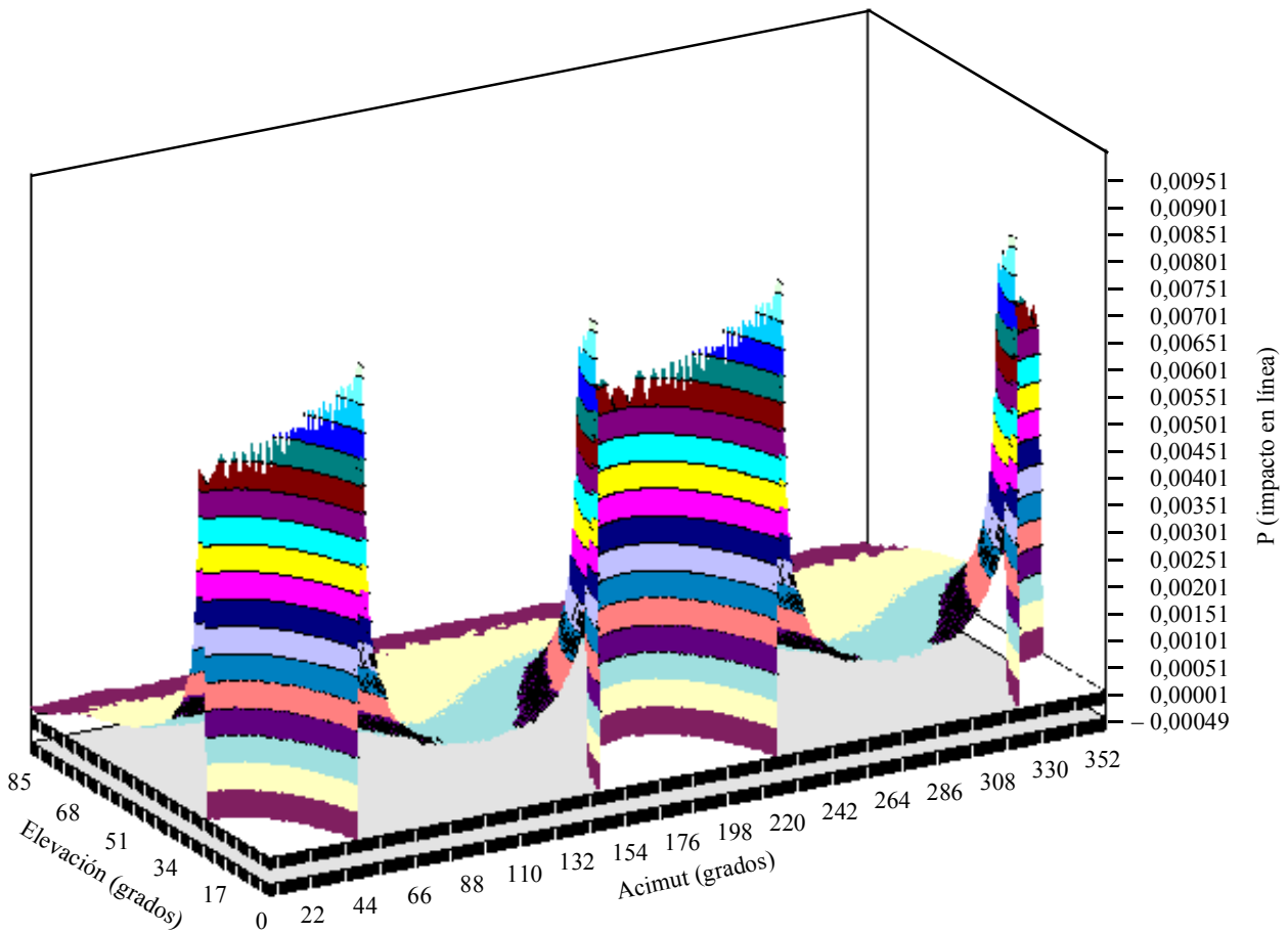
FIGURA 6a Valores estadísticos en línea para distintas direcciones de puntería: caso LEO-F, L_0 = 0^\circ , tamaño del haz = 3^\circ
