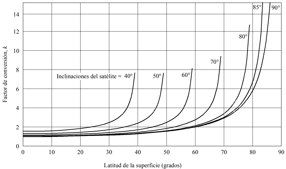
FIGURA 4 Factores de conversión para distintas inclinaciones y latitudes de la superficie
