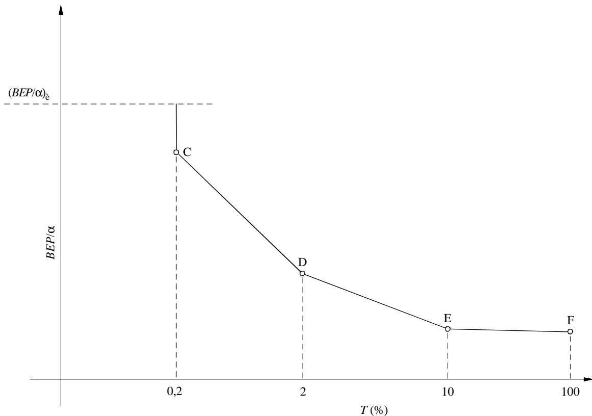
FIGURE 3 Gabarit simplifié
