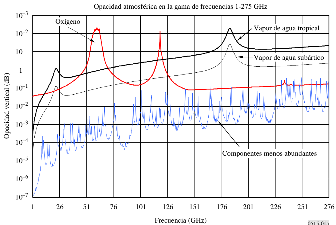
FIGURA 1a Atenuación en dirección del cenit en función de la frecuencia, 1-275 GHz
