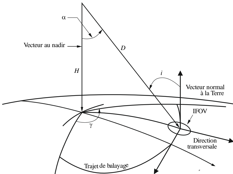
FIGURE 1 Configuration de balayage type d'un diffusiomètre à exploration conique
