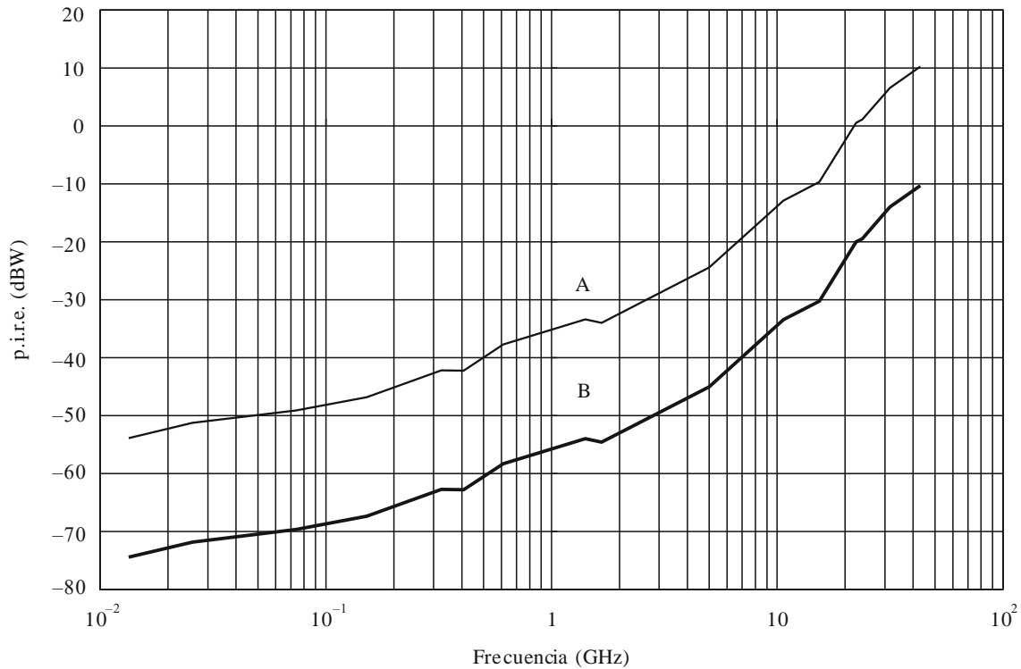
FIGURA 2 p.i.r.e. en función de la frecuencia
