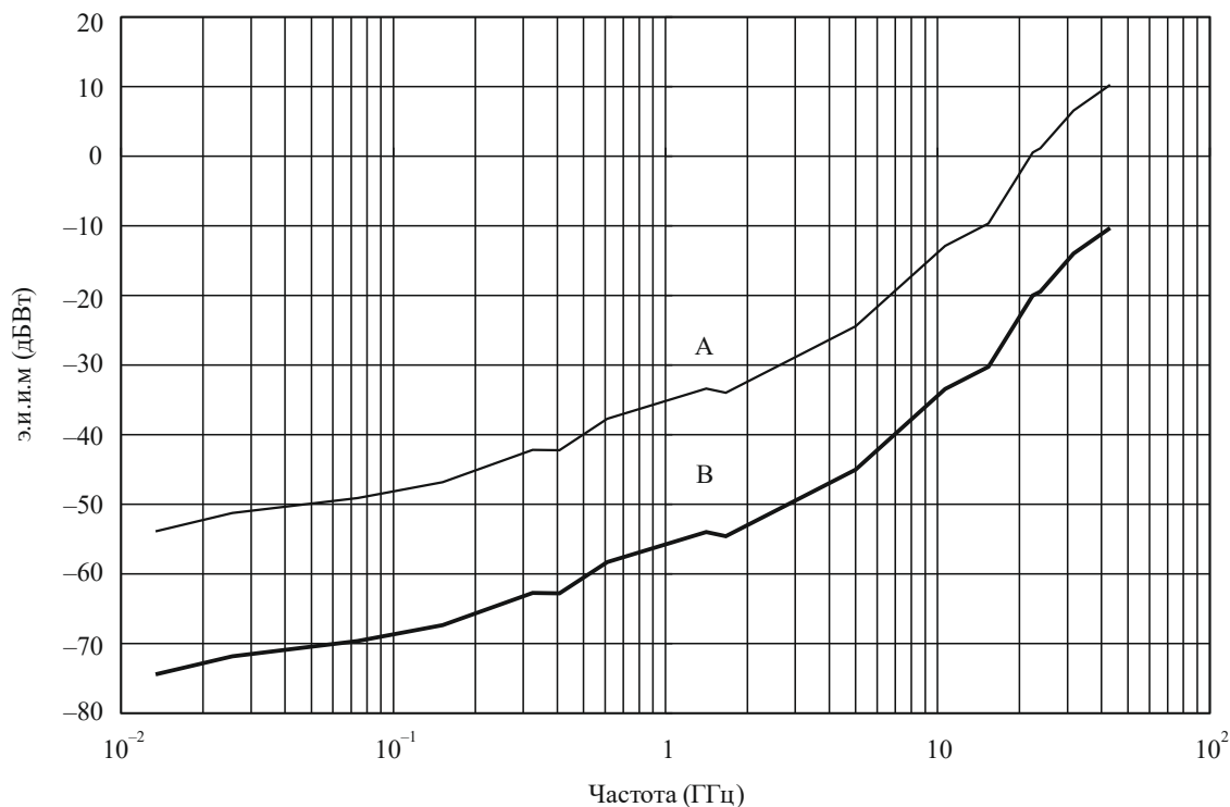
РИСУНОК 2 Э.и.и.м. как функция частоты
