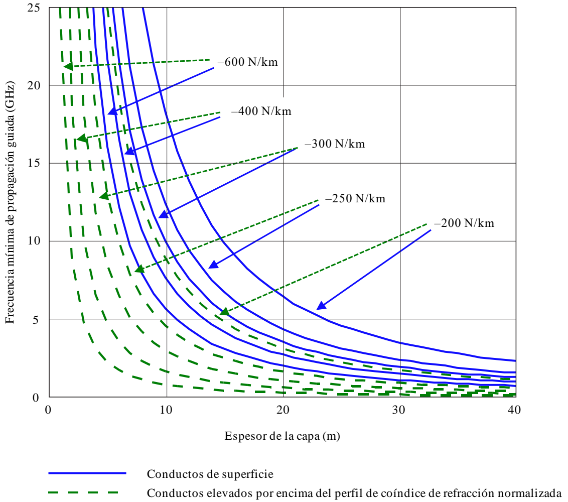
FIGURA 3 Frecuencia mínima de propagación guiada para conductos radioeléctricos atmosféricos de gradiente de coíndice constante
