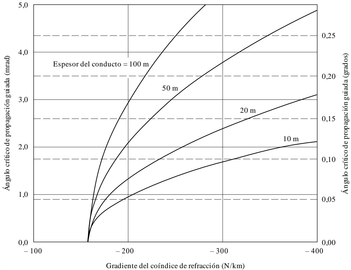
FIGURA 2 Ángulo máximo de propagación guiada para un conducto de superficie de gradiente de índice constante sobre una Tierra esférica
