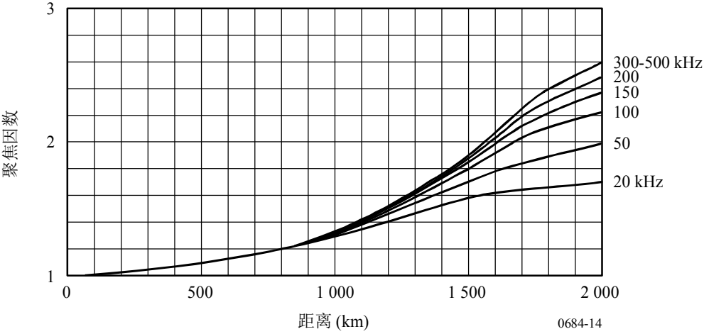
图 14 聚焦因数
