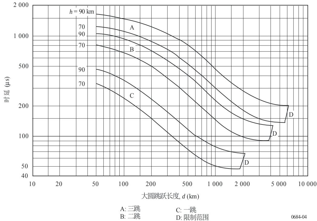
图 4 表面波和一跳、二跳或三跳天波之间的差分时延
