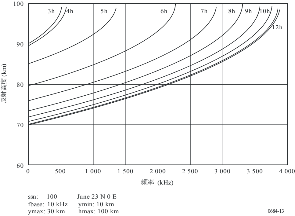
图 13 反射层的h-f曲线
