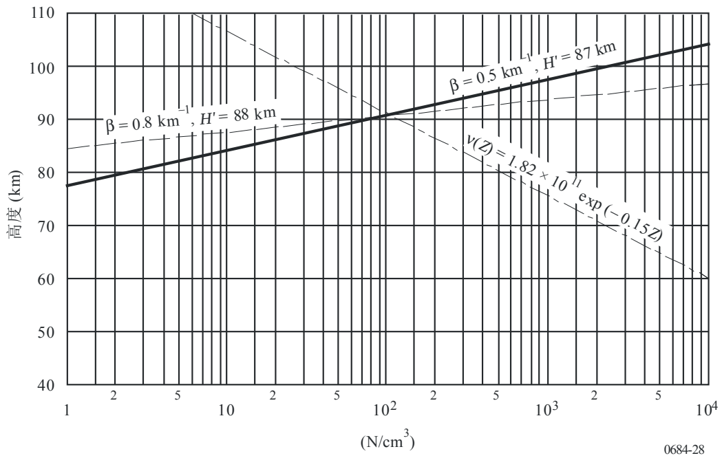
图 28 夜间电子密度分布和碰撞频率分布
