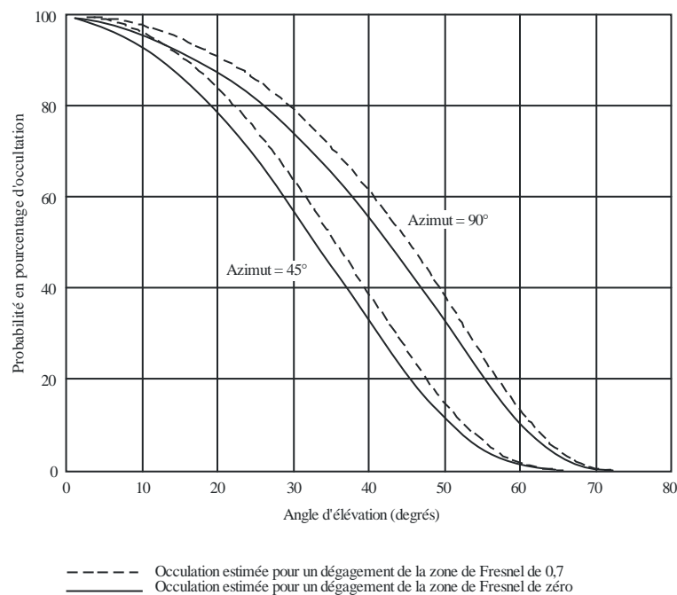
FIGURE 4 Exemples d'effet d'écran dû aux bâtiments construits en bordure des routes (voir le texte pour les valeurs des paramètres)
