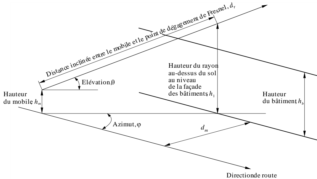
Géométrie du modèle d'effet d'écran dû aux bâtiments construits en bordure des routes
