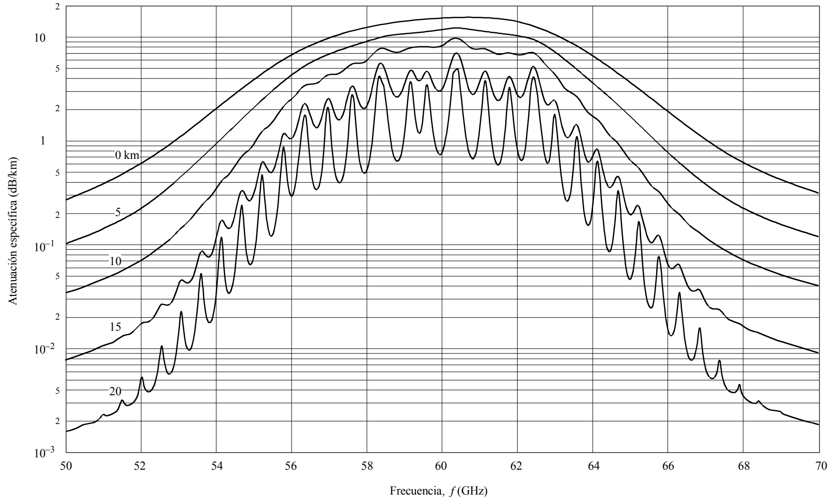
Atenuación específica en la gama de 50-70 GHz a las alturas indicadas
