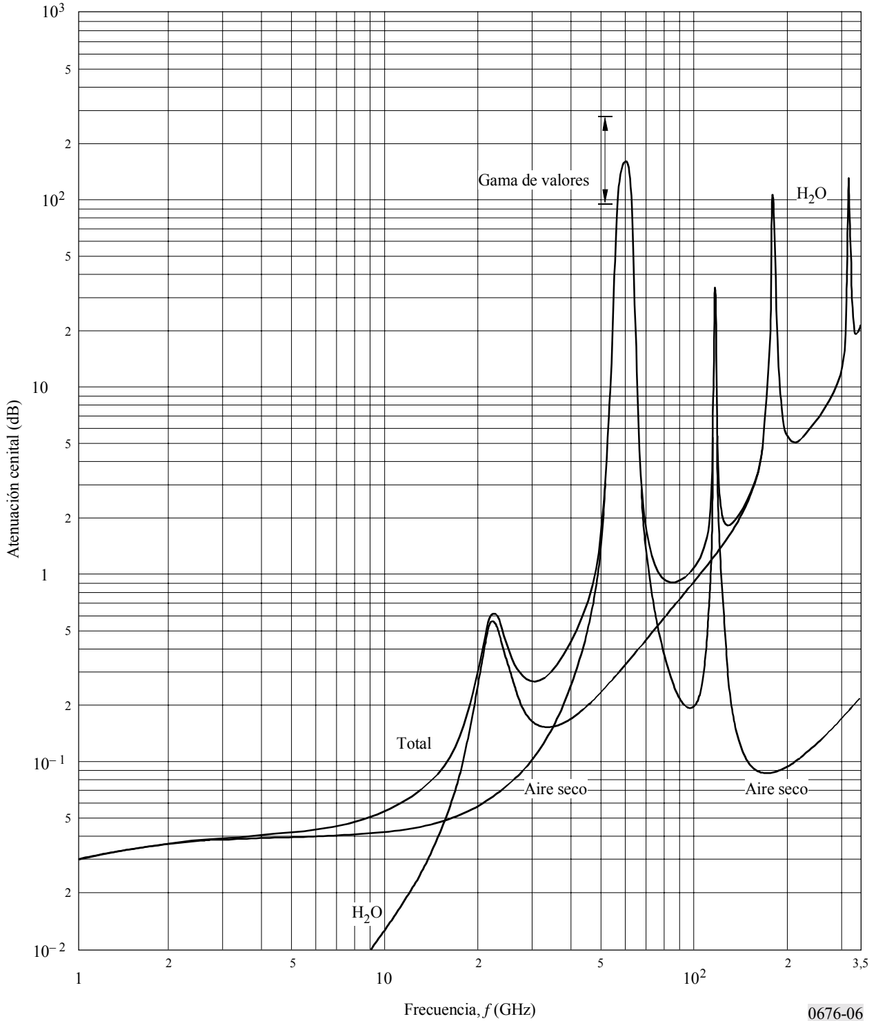
FIGURA 6 Atenuación cenital total a nivel del mar debida a la atmósfera seca y al vapor de agua
