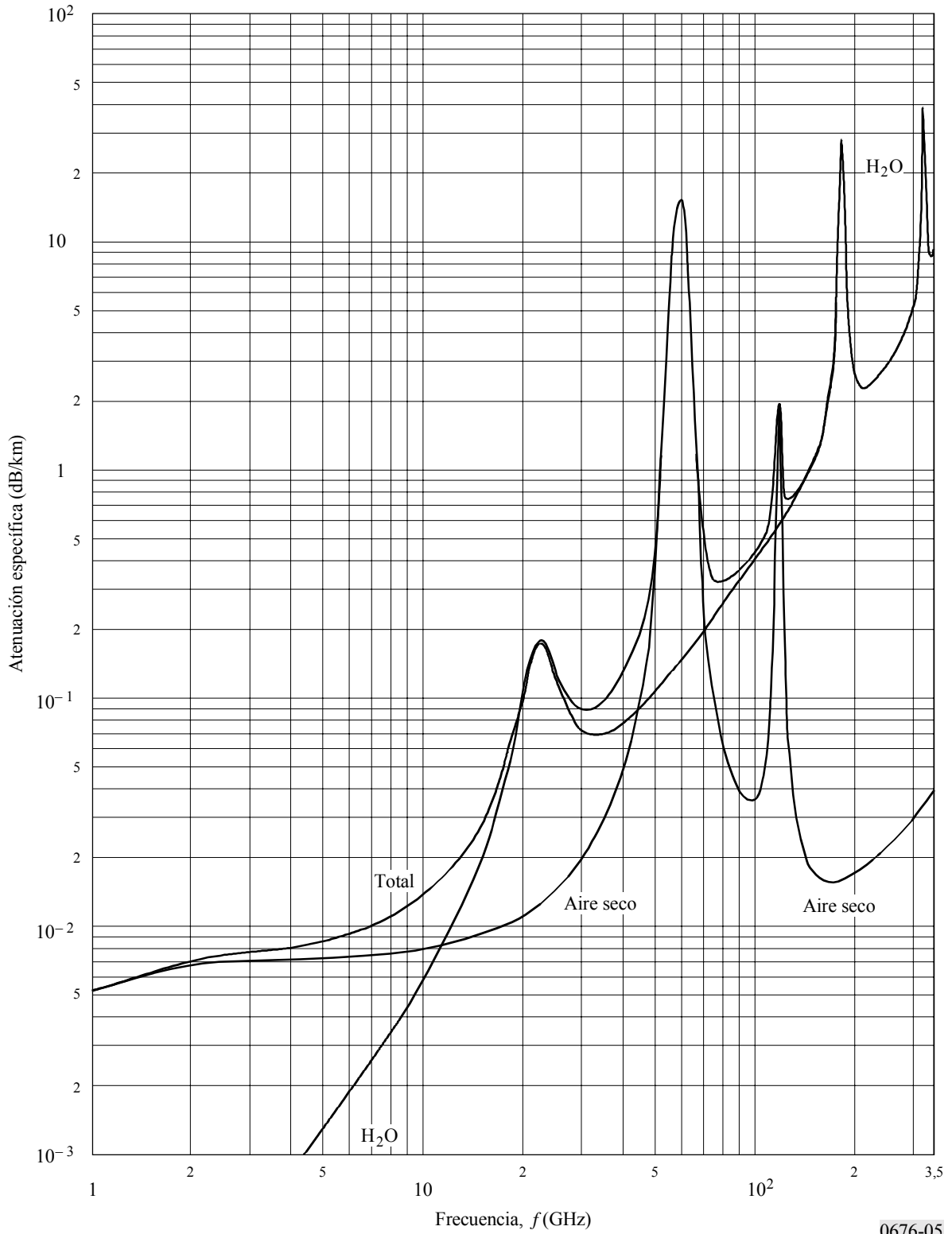
FIGURA 5 Atenuación específica debida a los gases atmosféricos
