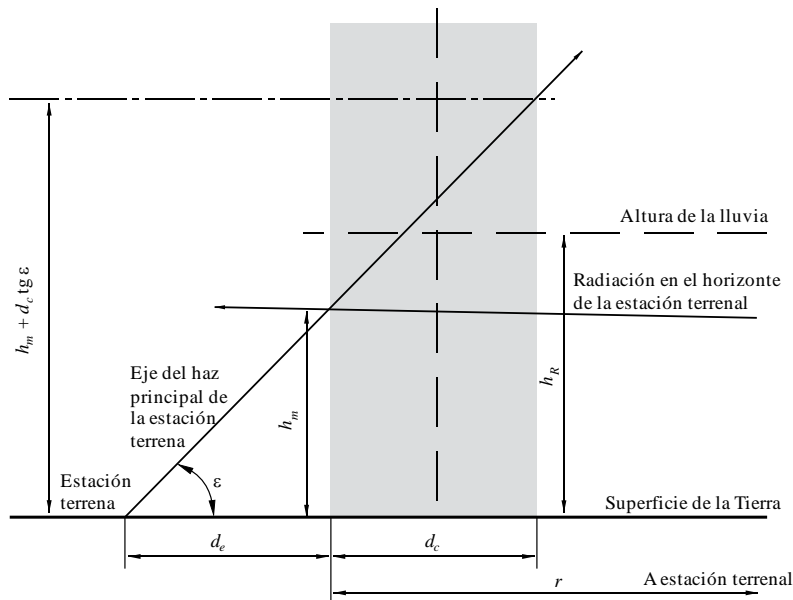
FIGURA 1 Geometría del proceso de dispersión debida a la lluvia
