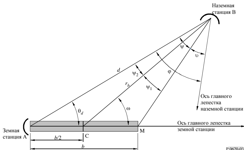
РИСУНОК 3 Геометрия распространения в горизонтальной плоскости
