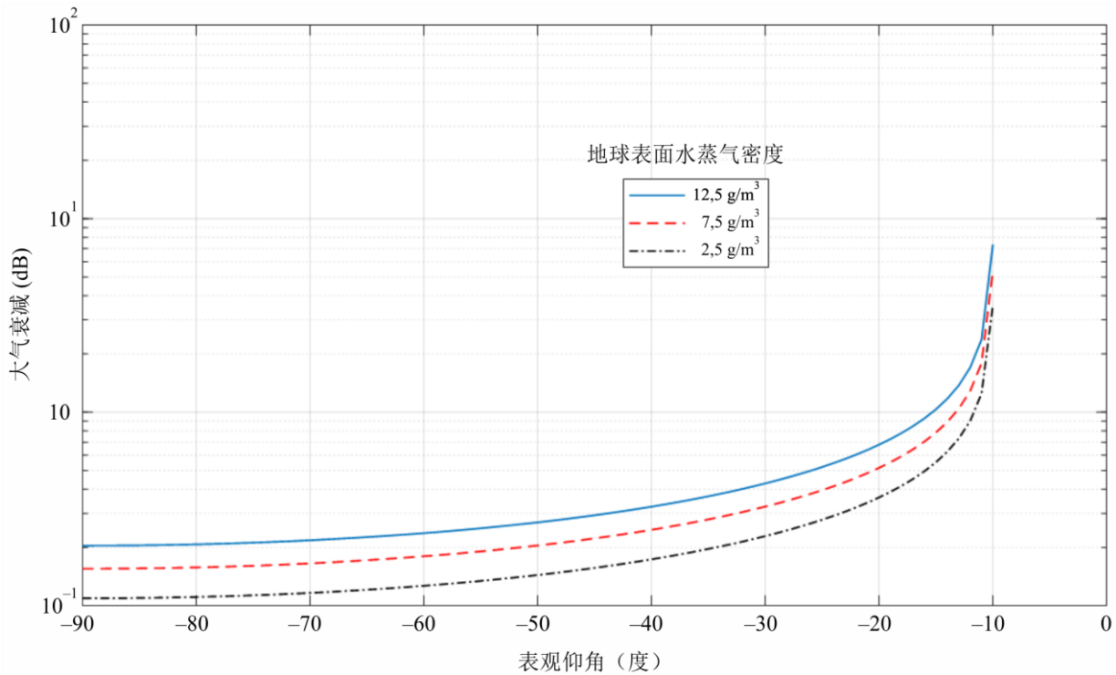
图4 沿空-地传播路径的大气衰减与仰角的关系 (空间电台海拔高度=100 km, 地球站海拔高度=1 km, 频率=30 GHz)
