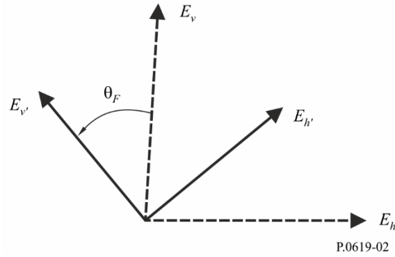
图2 垂直于传播方向的平面内法拉第旋转
