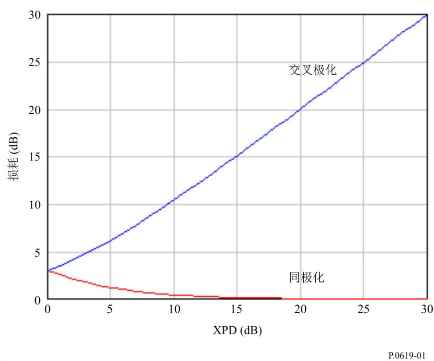
图1 同极化和交叉极化损耗与XPD的关系
