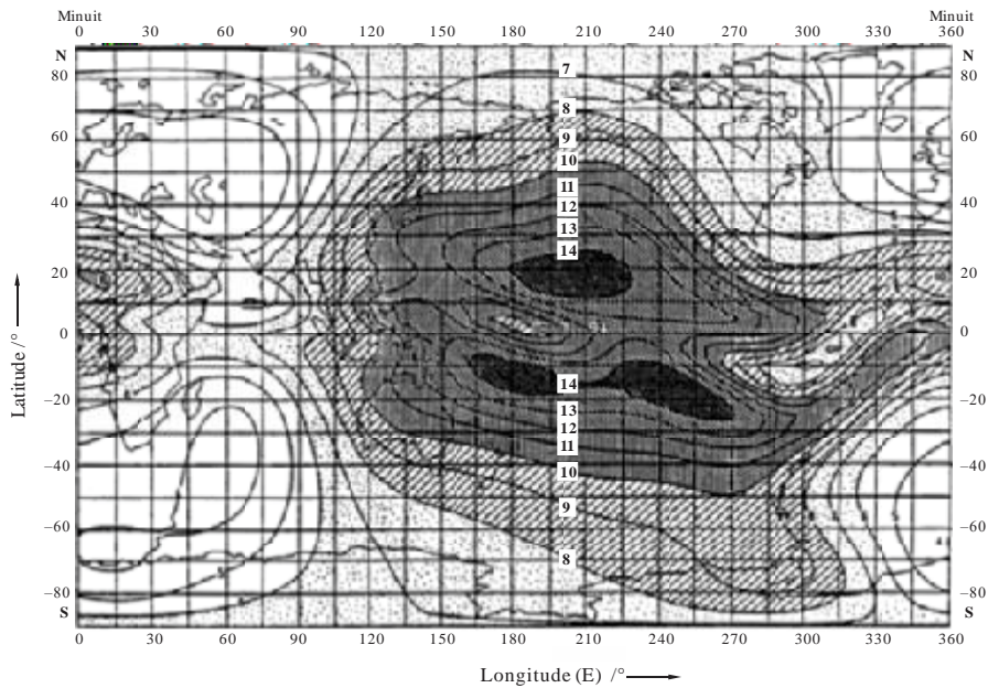
FIGURE 7 Réfraction ionosphérique
