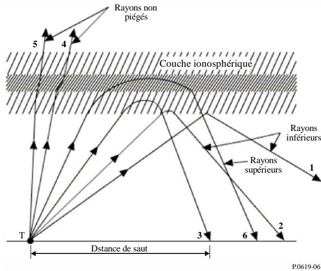
FIGURE 6 Réfraction ionosphérique
