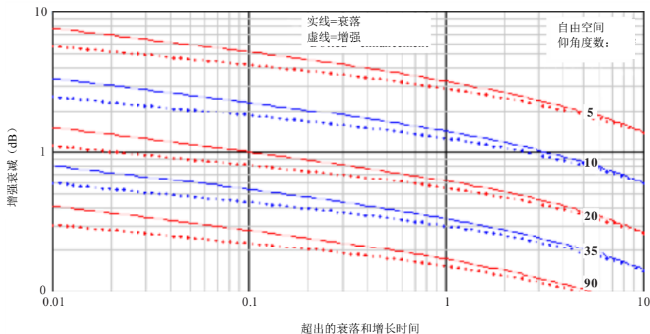
空间闪烁增强和衰落与自由空间仰角关系图 频率为30GHz, N_{wet} = 42.5 , 天线增益=0 dBi
