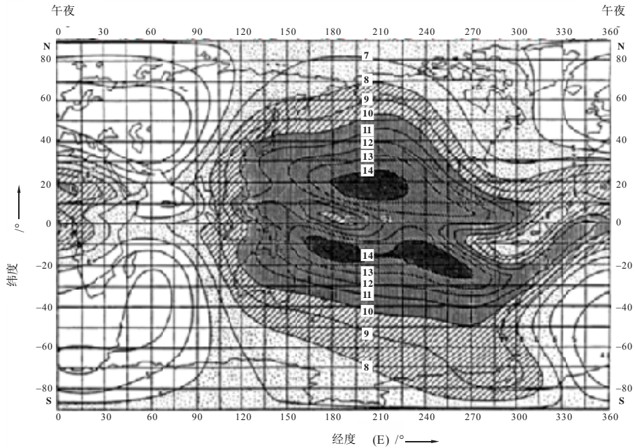
图6 电离层折射
