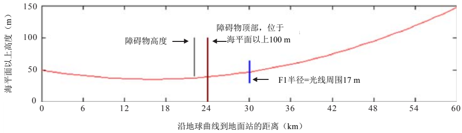
与地对空射线有关的衍射参数几何
