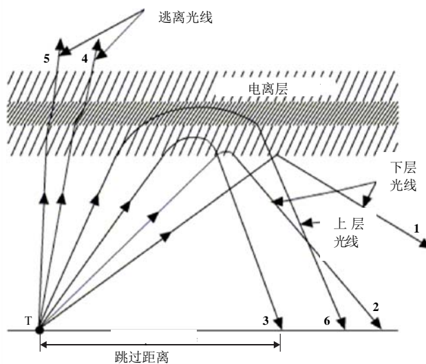
图5 电离层折射
