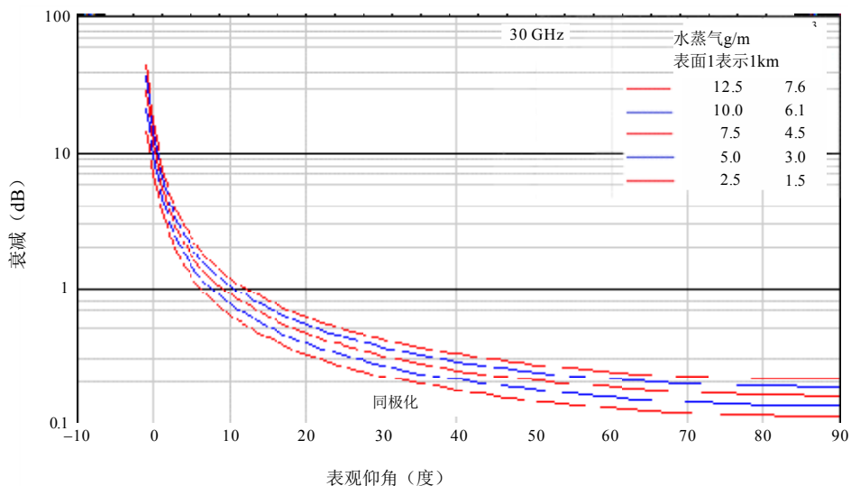
图3 气体吸收造成的衰减与仰角的关系曲线
