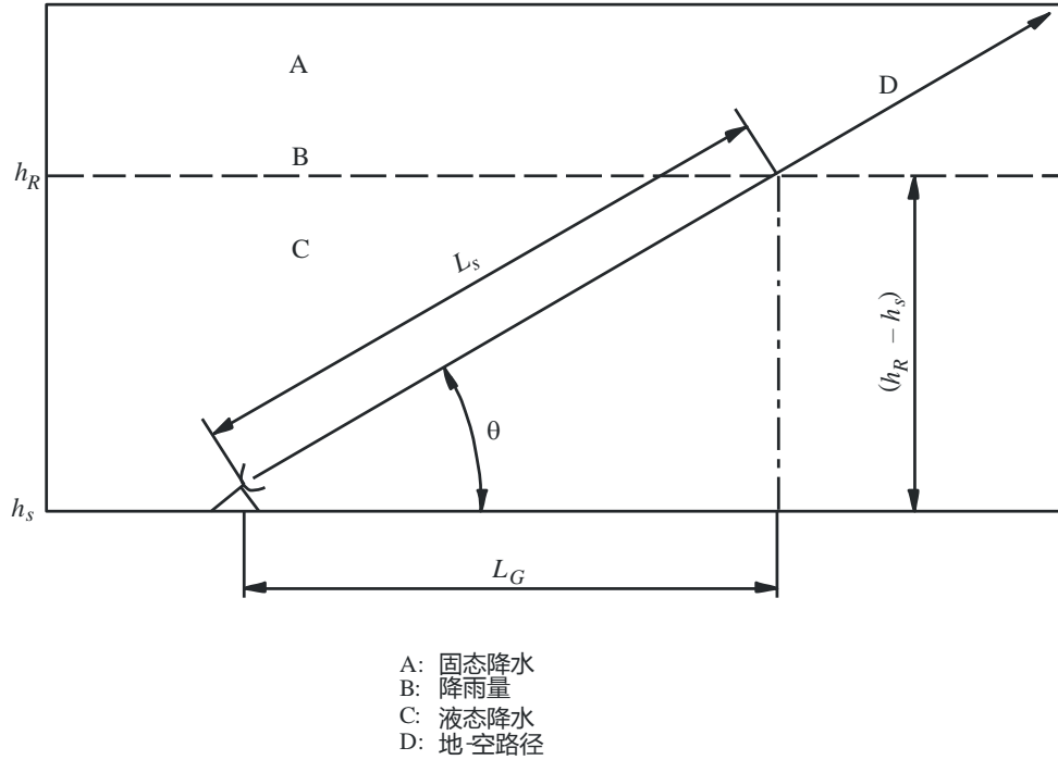
地-空路径上给定衰减预测过程输入参数的示意图
