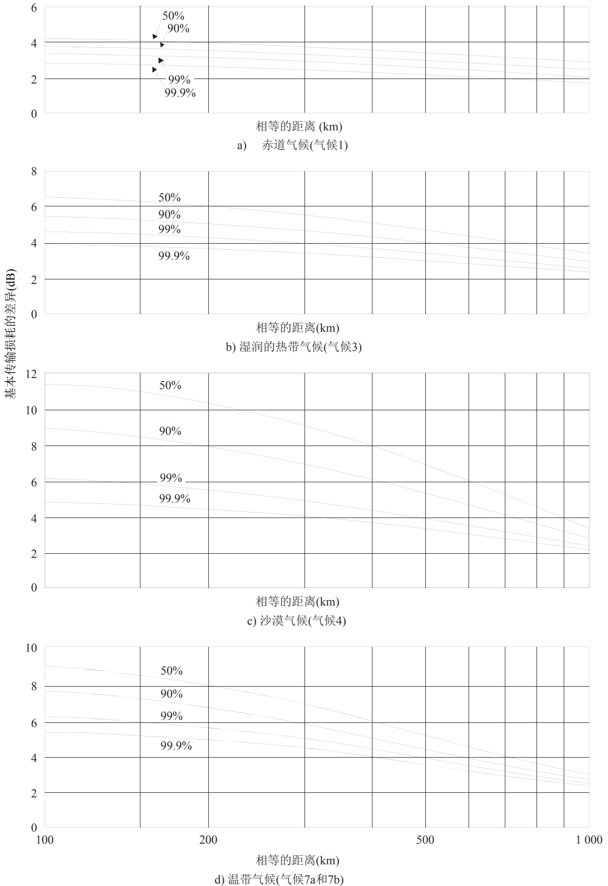
最坏月份基本传输损耗与年基本传输损耗的差异曲线
