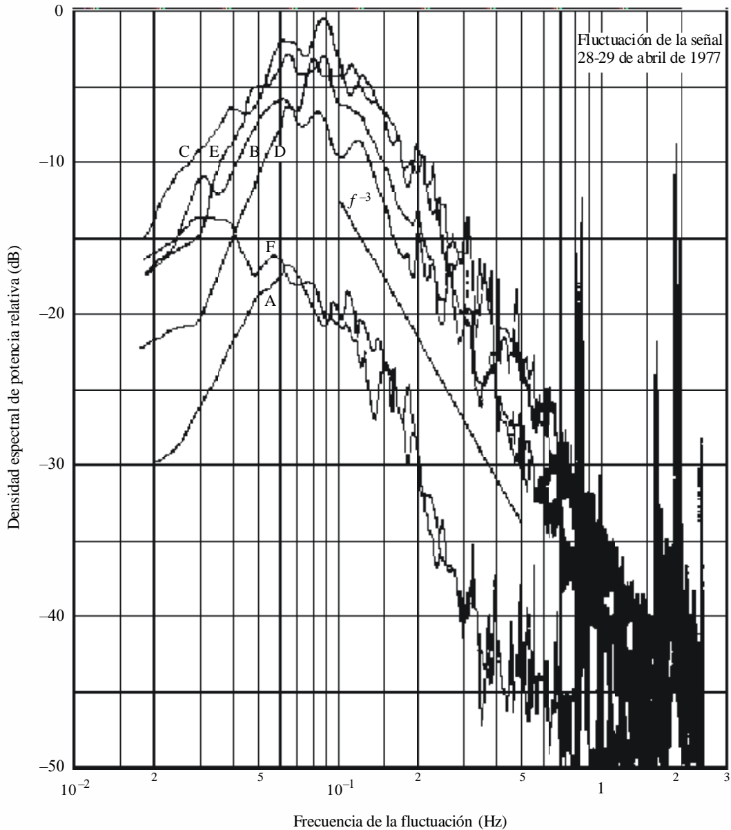
FIGURA 8 Estimaciones de la densidad espectral de potencia para un satélite geoestacionario (Intelsat-IV) en 4 GHz
