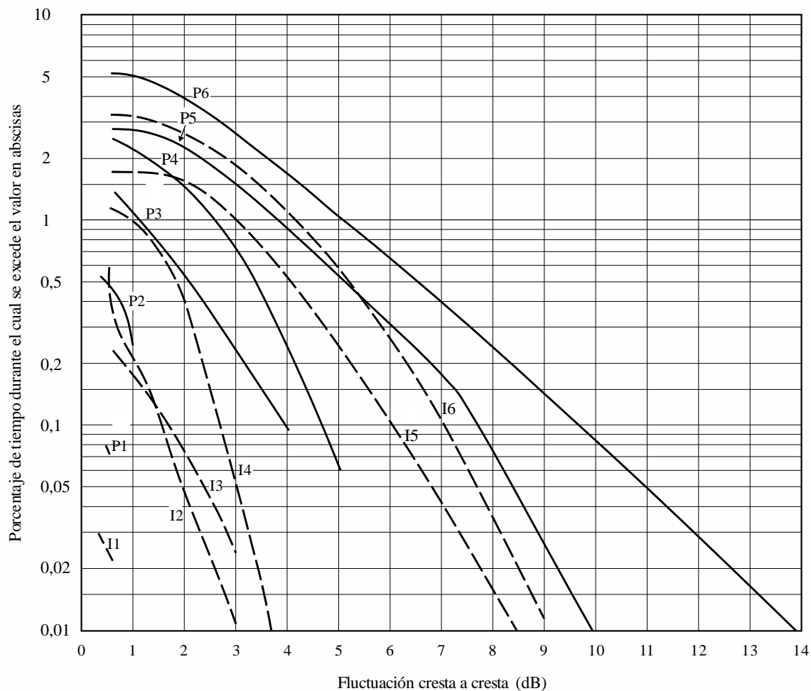
FIGURA 14 Valores estadísticos anuales de las fluctuaciones cresta a cresta observadas en la estación terrena de Hong Kong (curvas I1, P1, I3-I6, P3-P6) y la estación terrena de Taipei (curvas P2 e I2)
