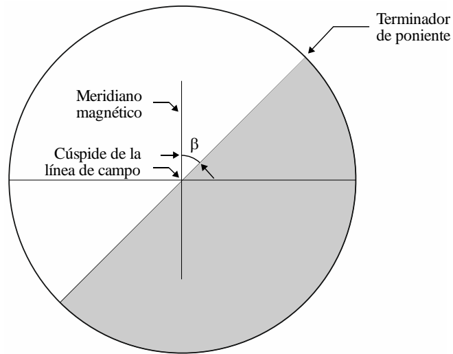
FIGURA 11 Ángulo comprendido entre el meridiano magnético local en la cúspide de la línea de campo indicada en la Fig. 10 y el terminador de poniente
