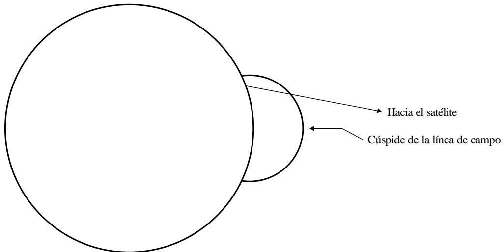
FIGURA 10 Intersección del trayecto de propagación con una línea de campo magnético a la altitud correspondiente a la región F
