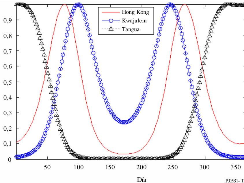
FIGURA 12 Funciones de ponderación estacionales correspondientes a estaciones de sectores de longitud diferentes
