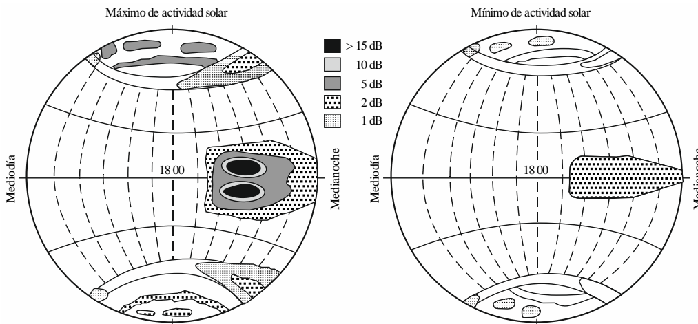
FIGURA 6 Intensidad del desvanecimiento por centelleo (proporcional a la densidad del sombreado) a 1,5 GHz durante los años de máxima y mínima actividad solar
