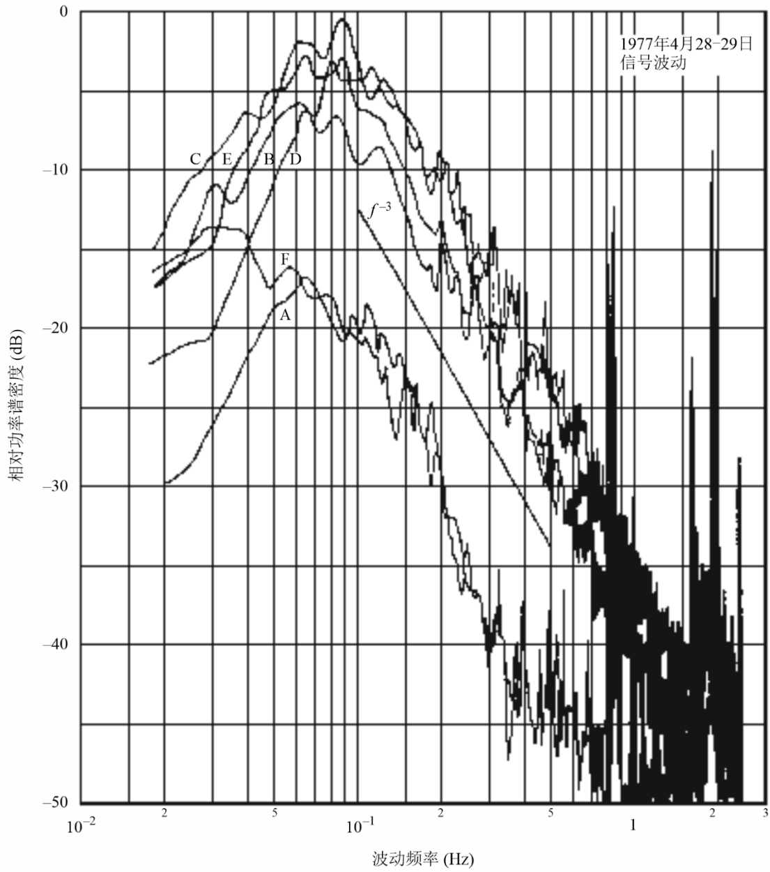
对地静止轨道卫星 (Intelsat-IV) 在4 GHz功率谱密度估计
