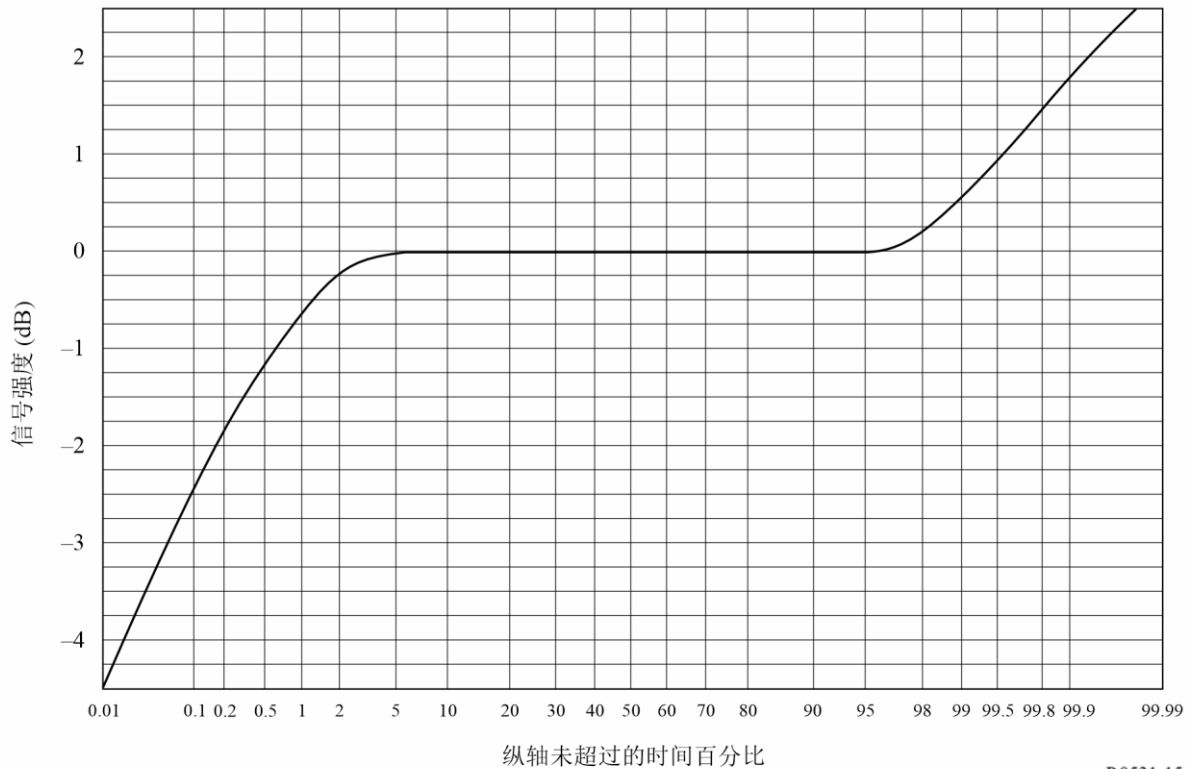
图15 信号强度长期累积统计示例（4 GHz，20°仰角）
