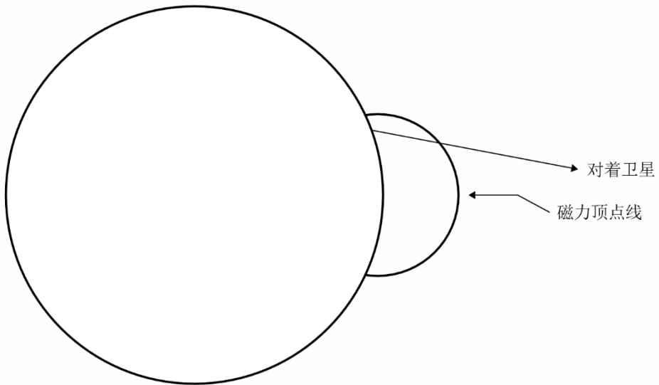
图10 F区域高度上传播路径和磁力线的交叉点
