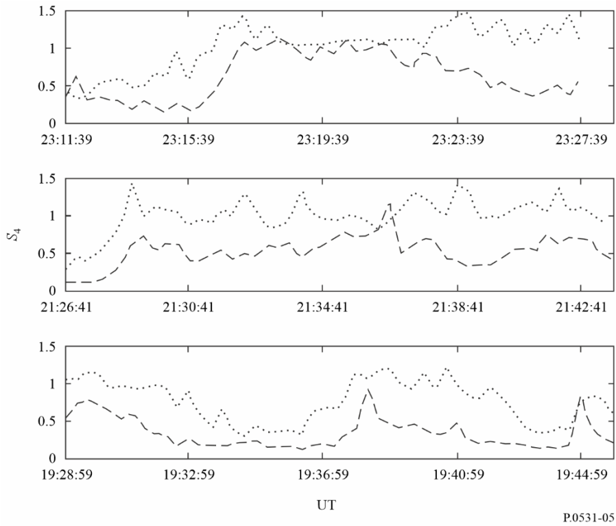
极轨LEO卫星Tsykada记录的2003年10月30日受扰情况下Kiruna (a)、Lulea (b)和Kokkola (c)站观测的150 MHz (点线)和400 MHz (短划线) 闪烁指数
