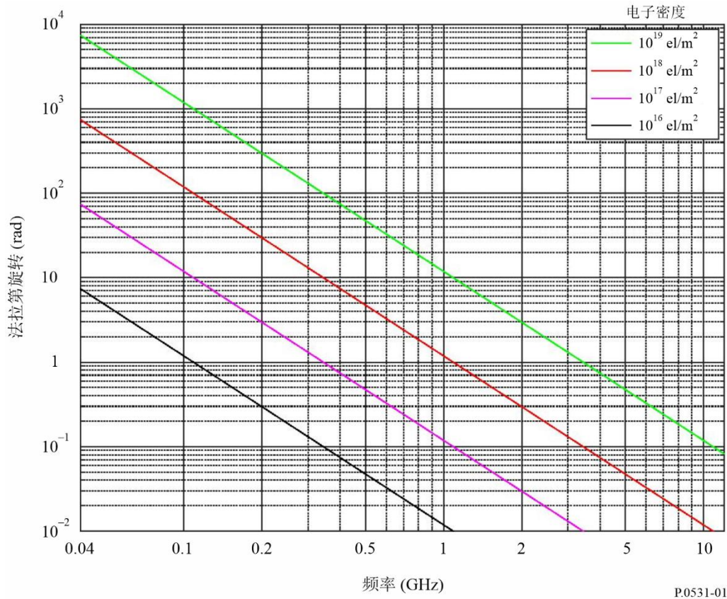
图1 法拉第旋转作为TEC和频率的函数
