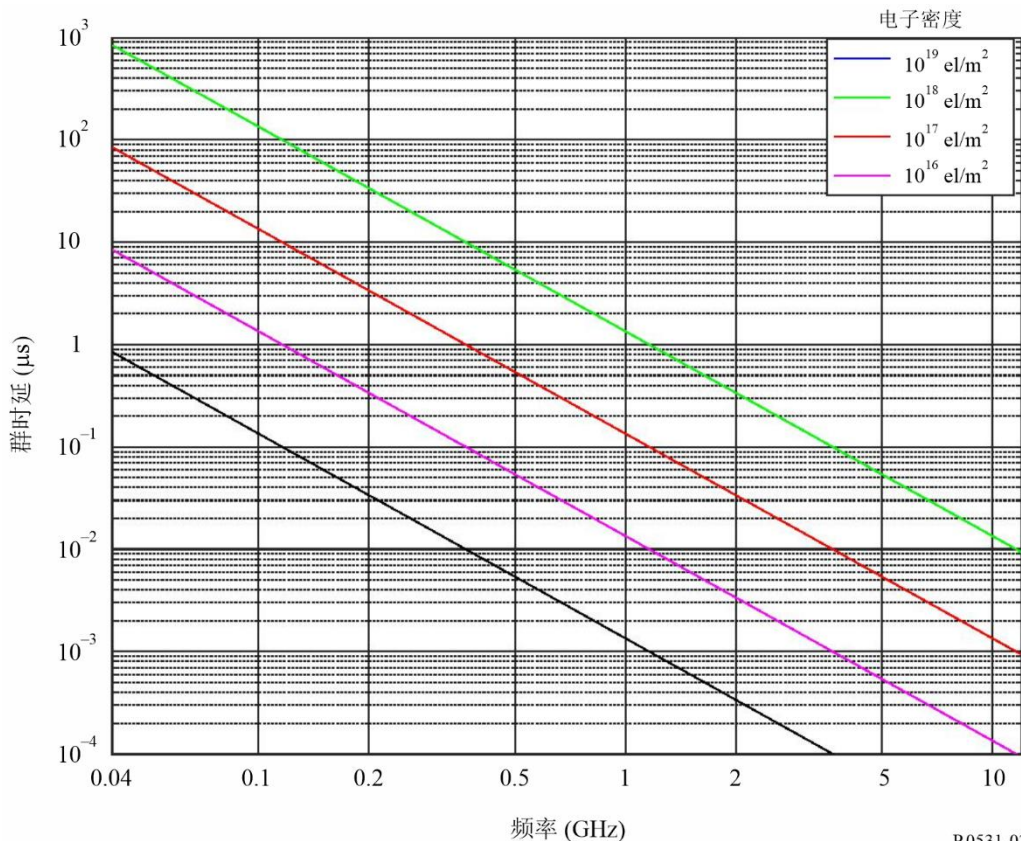
图2 不同电子容量时电离层时延和频率的关系
