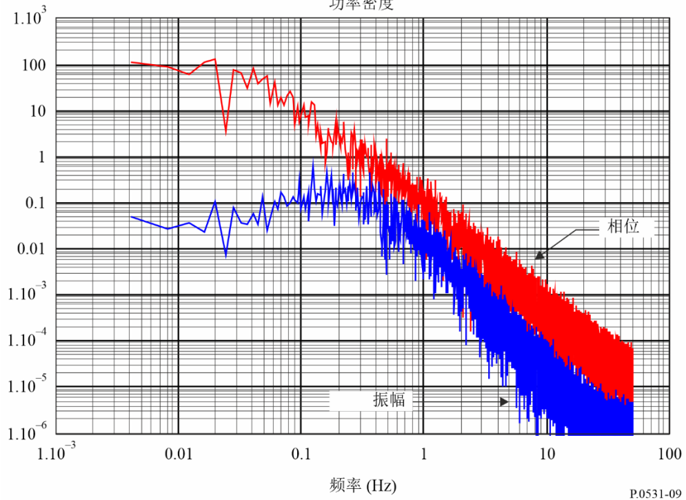
图9 典型强度和相位谱 功率密度
