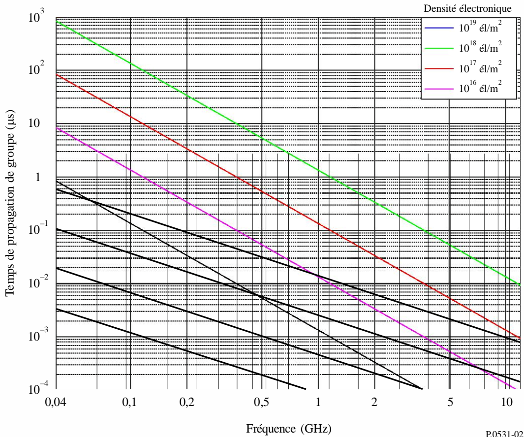
FIGURE 2 Temps de propagation de groupe dans l'ionosphère en fonction de la fréquence, pour diverses valeurs du contenu électronique
