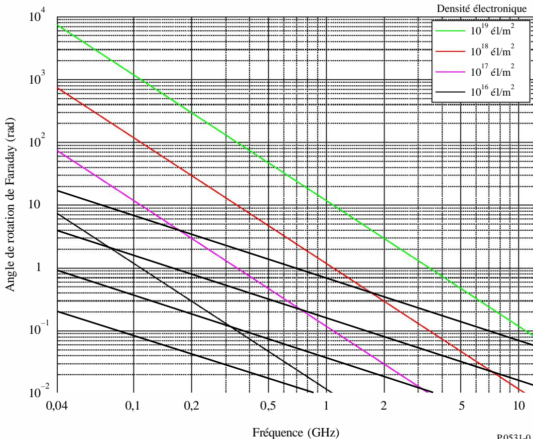
FIGURE 1 Rotation de Faraday en fonction du CET et de la fréquence
