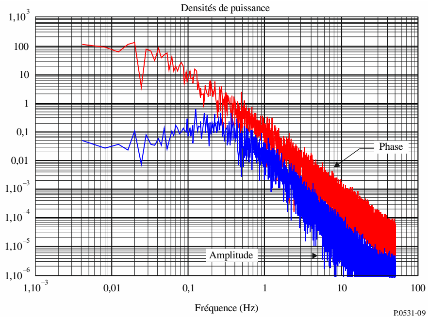
FIGURE 9 Spectres d'intensité et de phase typiques
