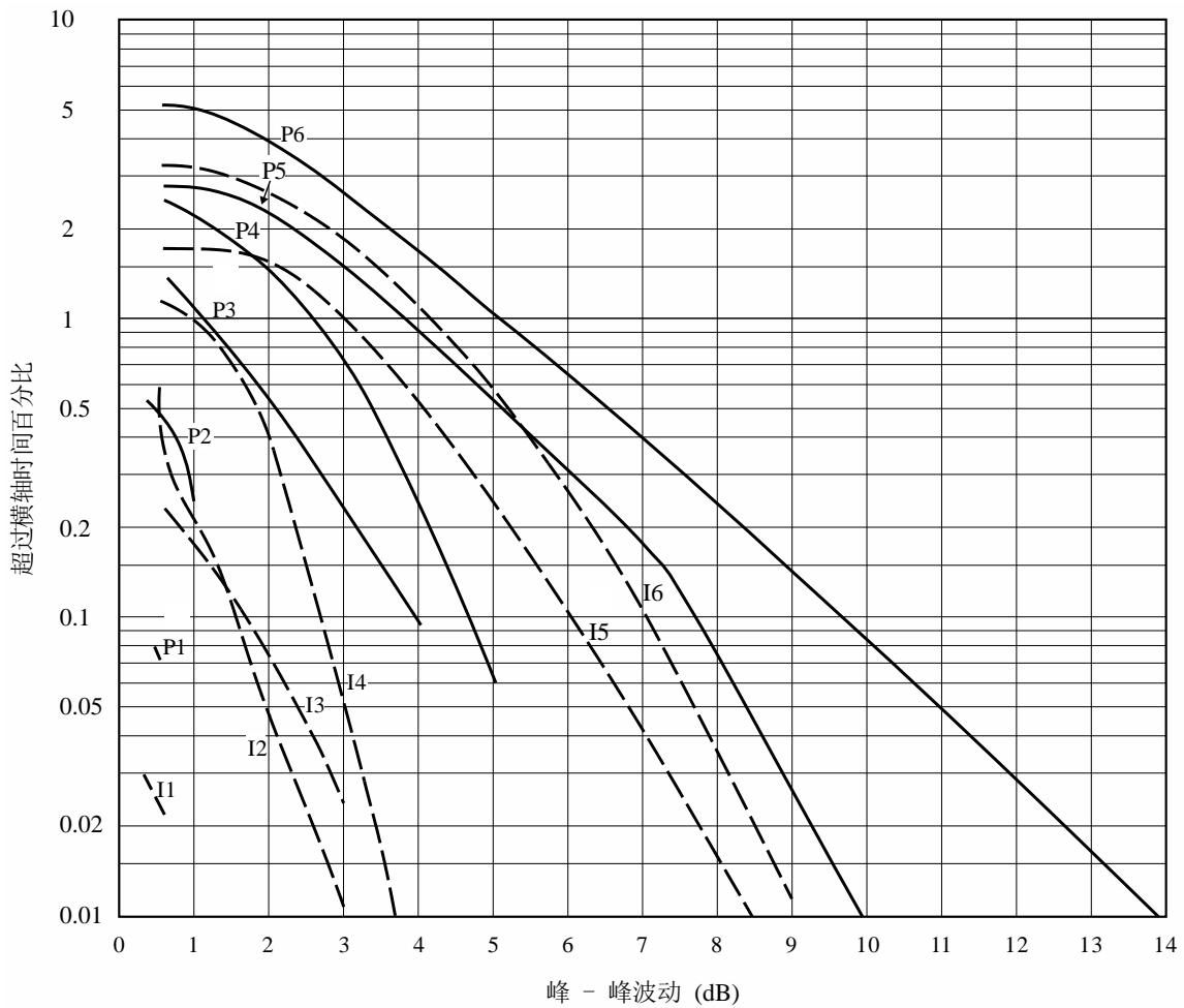
图12 中国香港地球站 (曲线I1, P1, I3-I6, P3-P6) 和中国台北地球站 (曲线P2和I2) 观测到的峰-峰波动值年统计表
