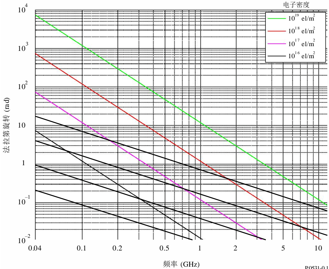
图1 法拉第旋转作为TEC和频率的函数
