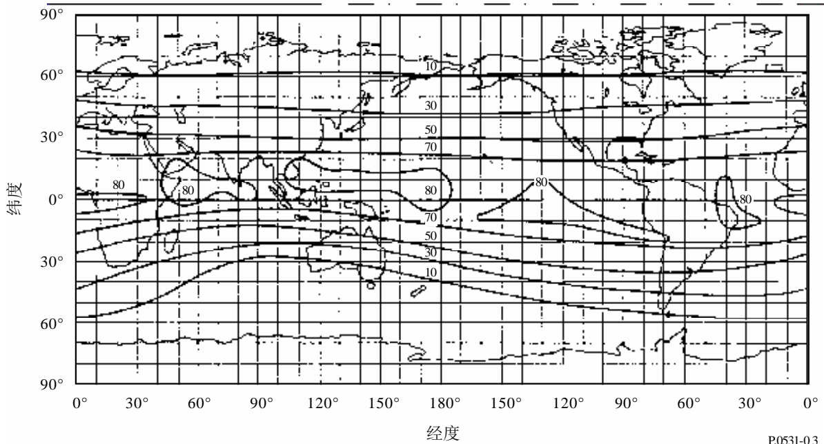
图3 1.6 GHz垂直入射情况下，时延超过20 ns的日间小时年平均百分比等值曲线（太阳黑子=140）
