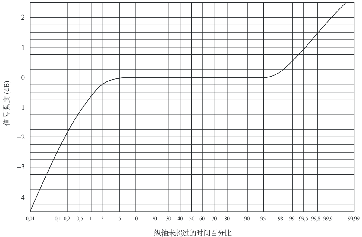
图13 信号强度长期累积统计示例 (4 GHz, 20°仰角)
