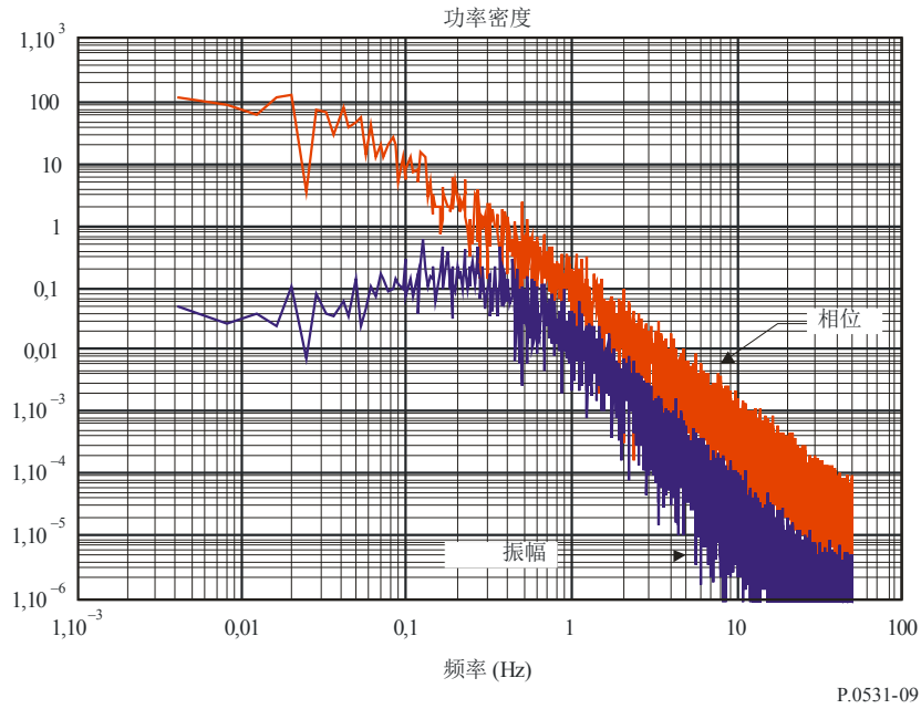
图9 典型强度和相位谱
