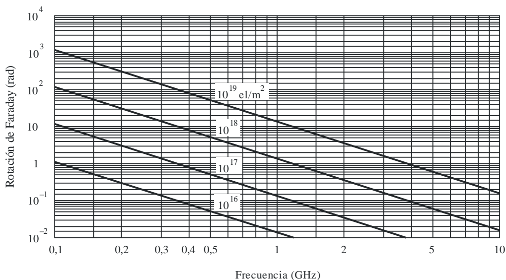
Rotación de Faraday en función del CET y de la frecuencia
