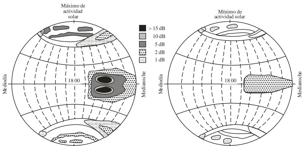
Intensidad del desvanecimiento por centelleo (proporcional a la densidad del sombreado) a 1,5 GHz durante los años de máxima y mínima actividad solar
