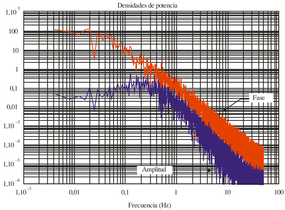
FIGURA 9 Espectro de intensidad y fase típico
