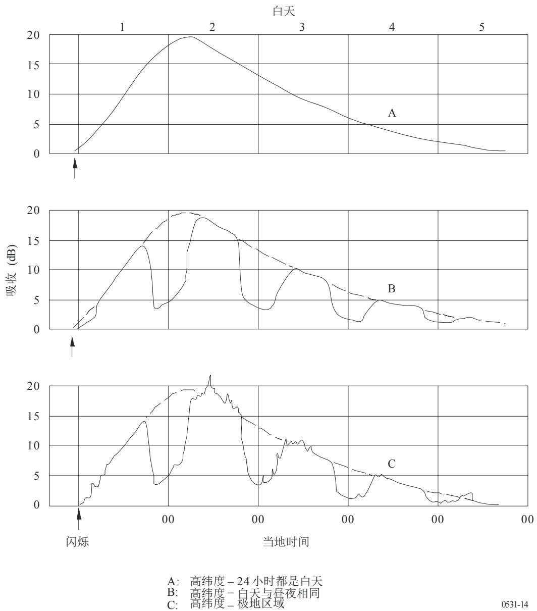
图14 发生严重太阳耀斑后期望通过电离层测定器在30 MHz 附近表现出的极冠吸收的假设模型
