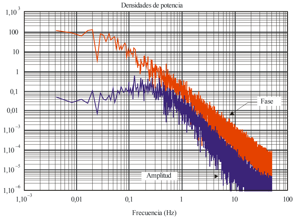
FIGURA 9 Espectro de intensidad y fase típico
