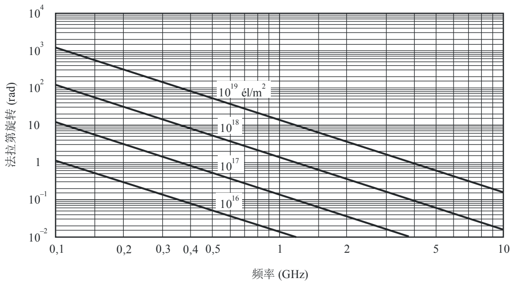
法拉第旋转作为TEC和频率的函数
