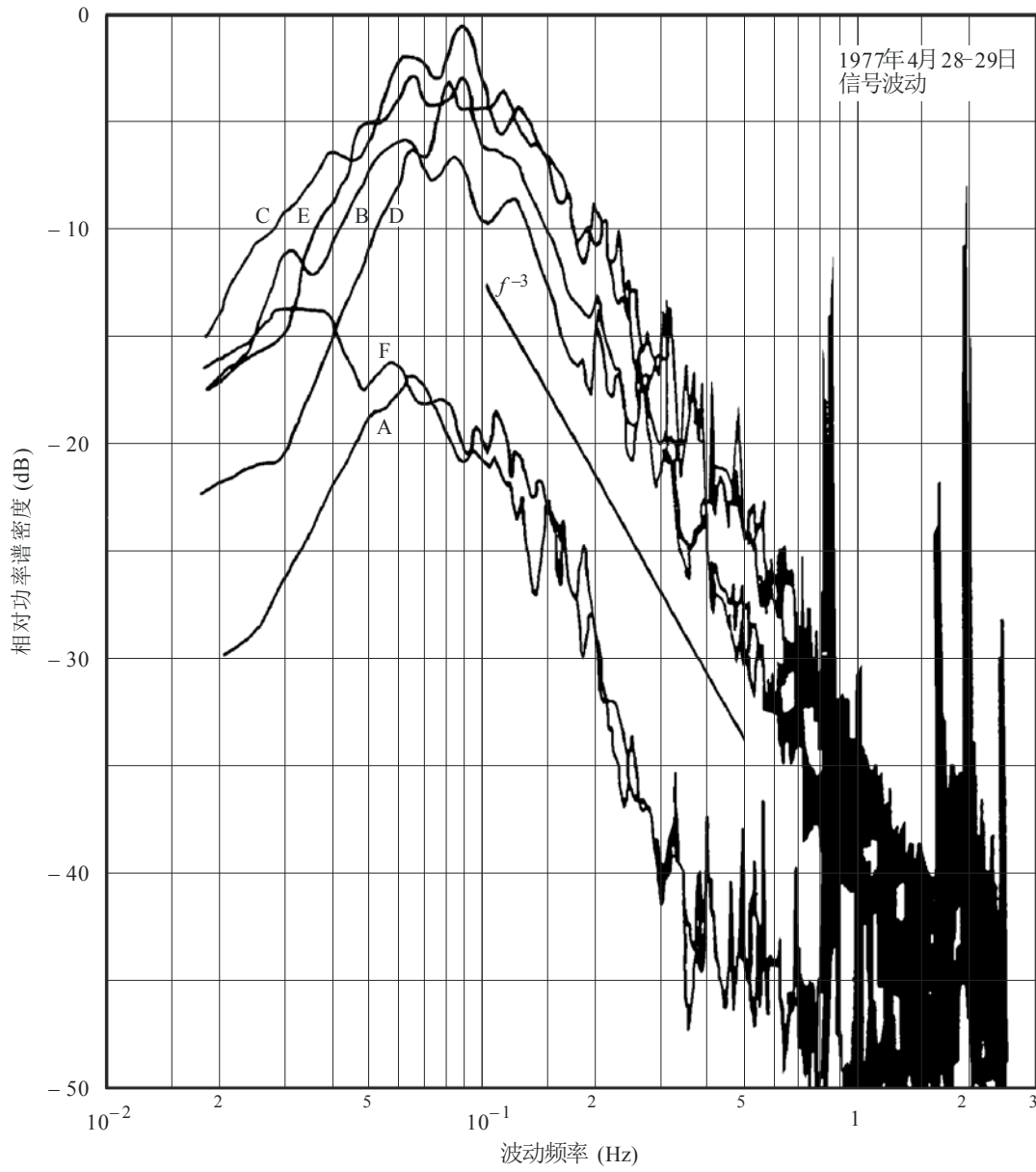
1977年4月28-29日傍晚中国台北 地球站观测到的闪烁事件
