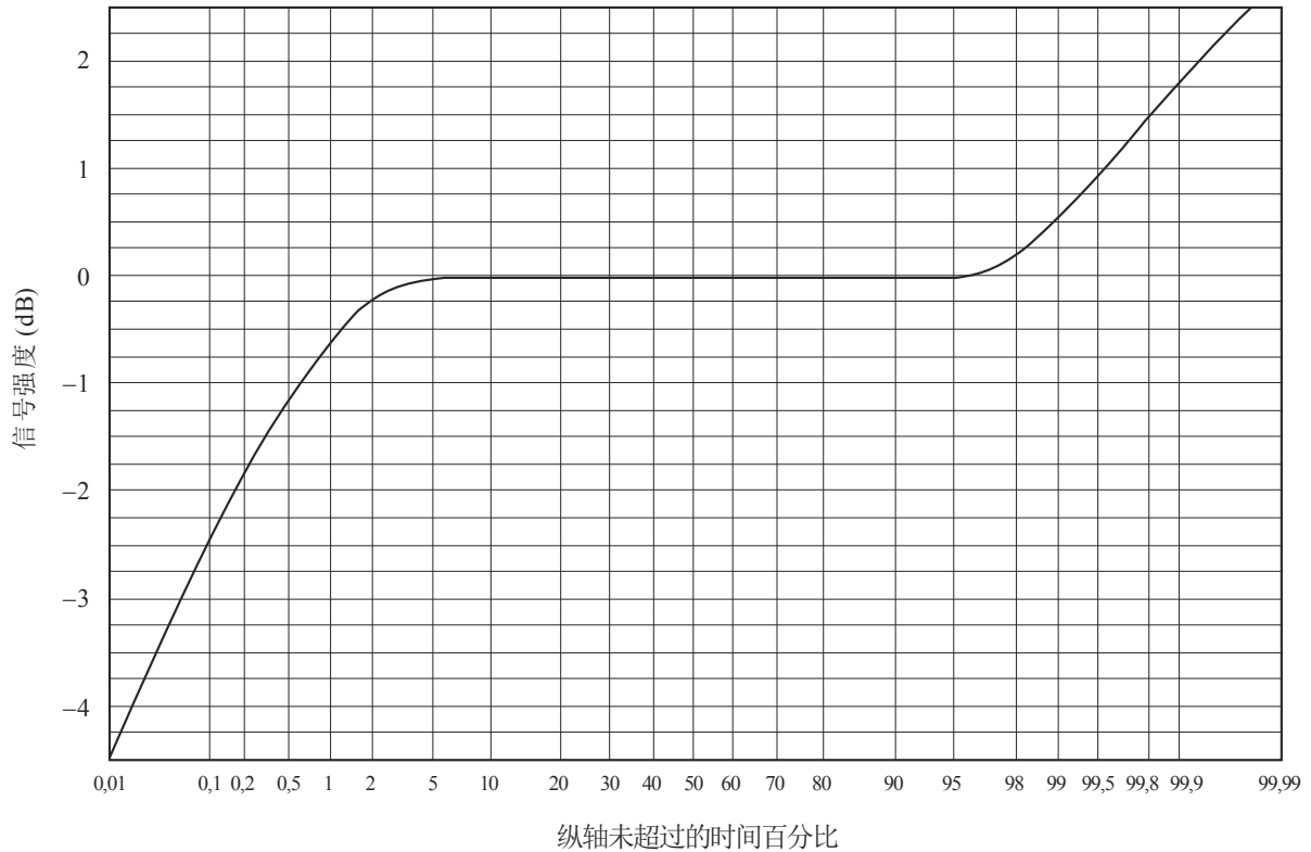
信号强度长期累积统计示例（4 GHz，20°仰角）
