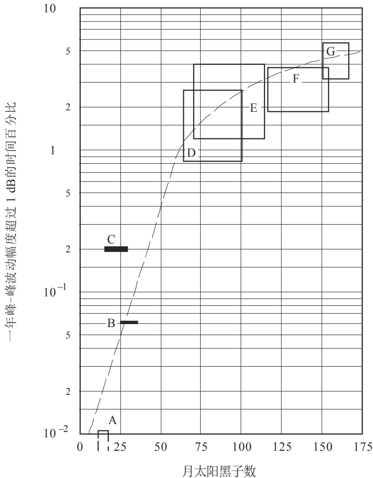
对应太阳黑子月平均数的4 GHz赤道电离层闪烁的关系曲线
