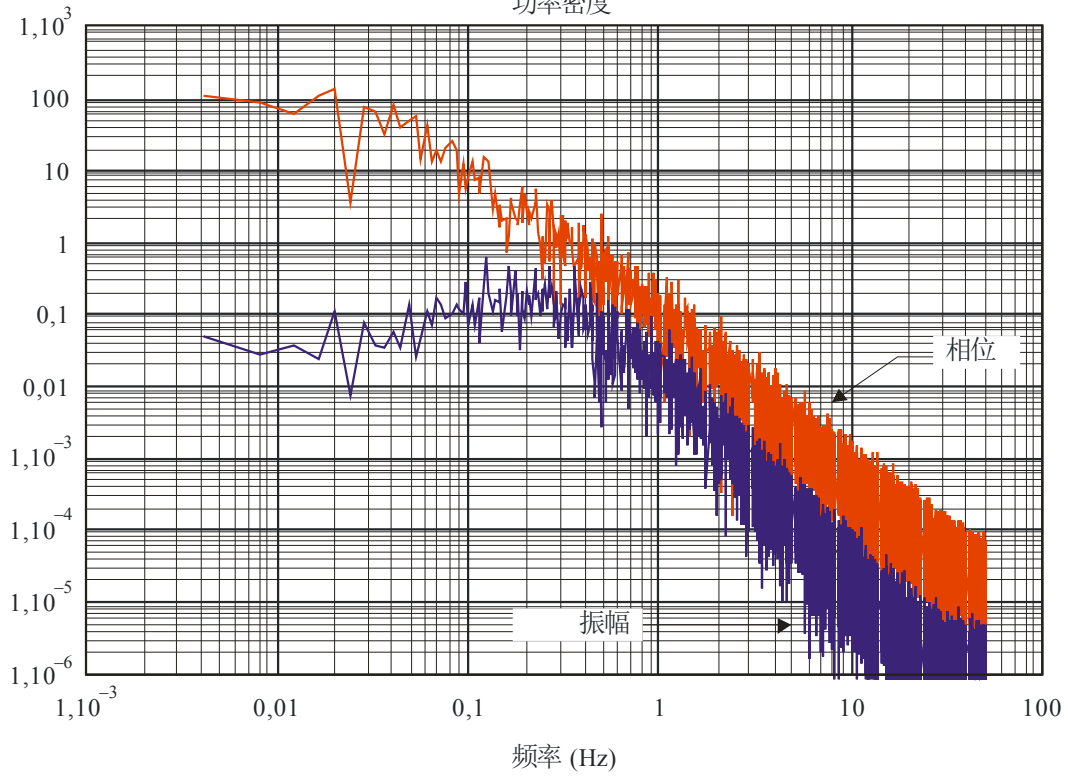
图9 典型强度和相位谱 功率密度
