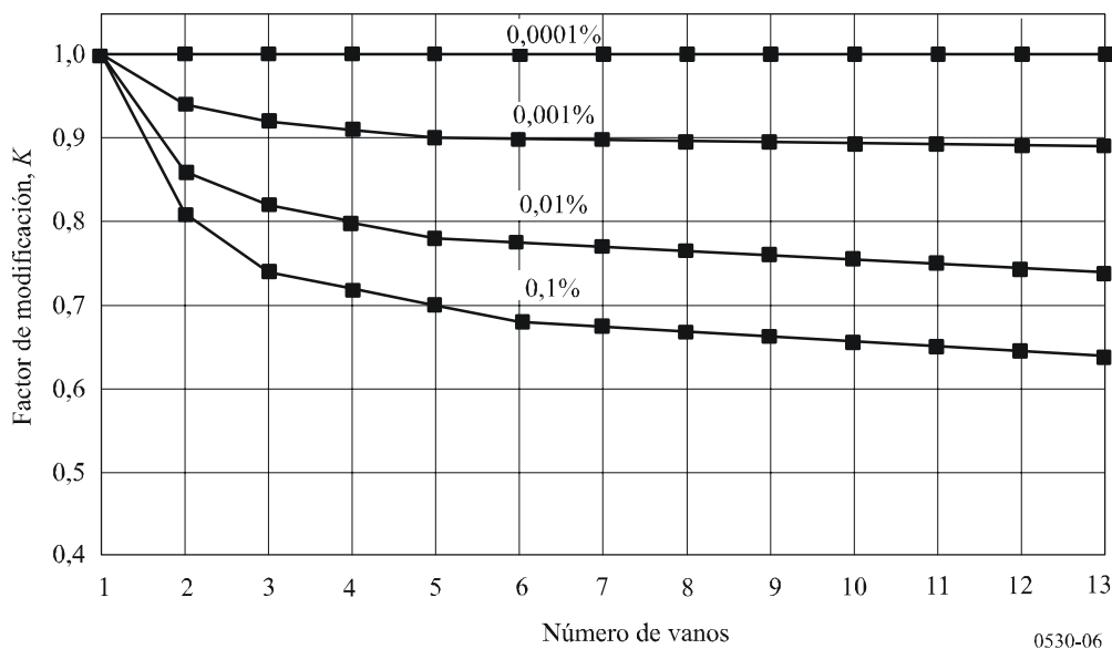
FIGURA 6 Factor de modificación de la atenuación total debida a la lluvia sobre una serie de vanos en tándem, cada uno de una longitud aproximada de 4,6 km, para varios niveles de probabilidad de excederse en cada enlace
