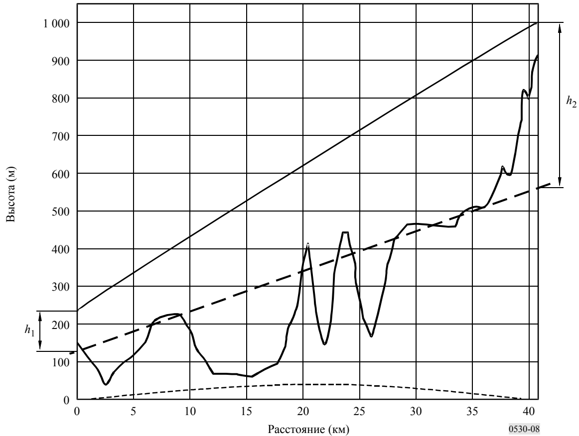
РИСУНОК 8 Трасса с отражающим рельефом местности
