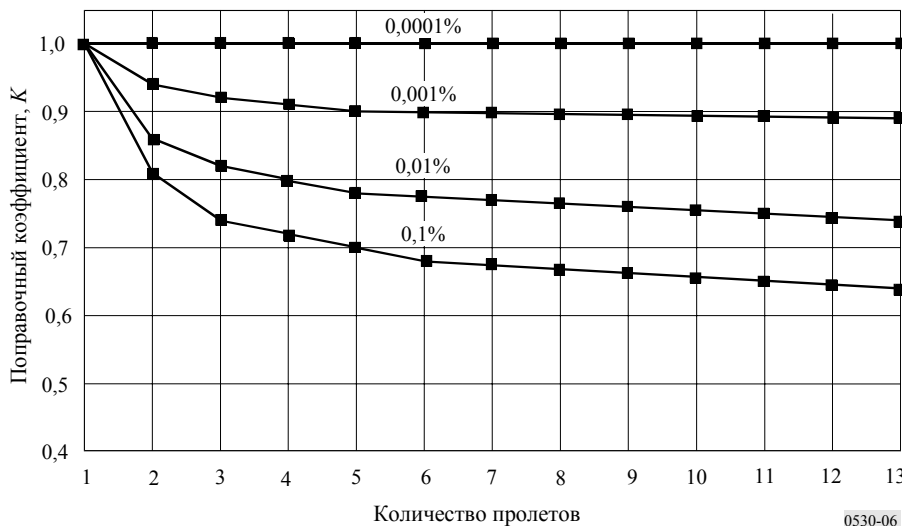
РИСУНОК 6 Поправочный коэффициент для общего затухания в дожде на серии последовательных пролетов длиной около 4,6 км каждый для различных уровней вероятности превышения на каждом пролете (май 1975 г. – март 1979 г.)
