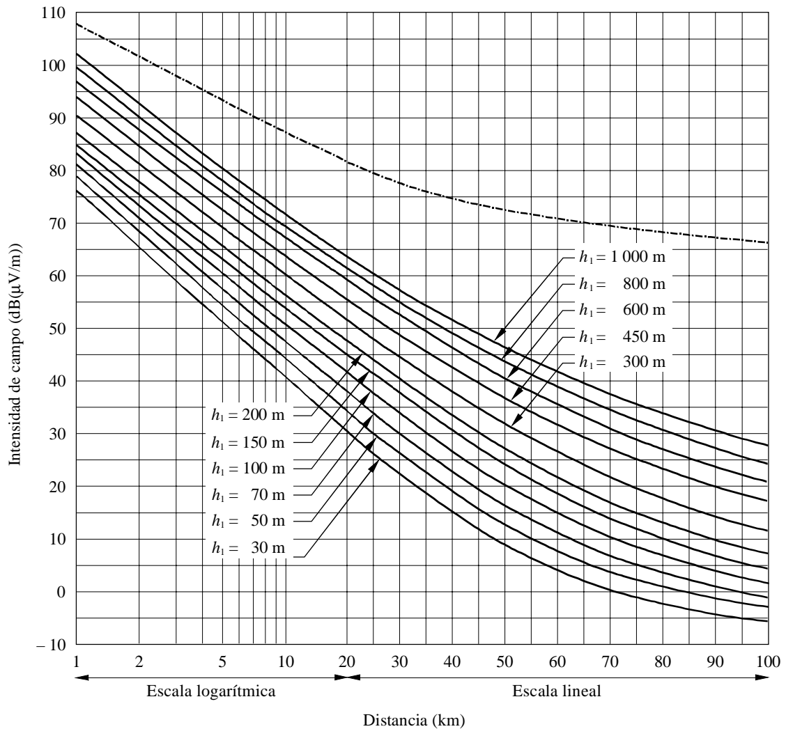
FIGURA 4 Intensidad de campo (dB(μV/m)) para 1 kW de potencia radiada aparente
