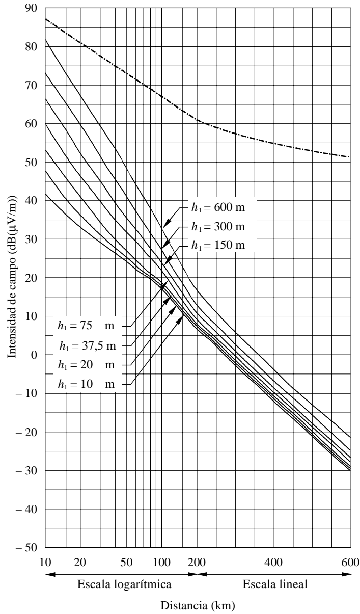
FIGURA 3 Intensidad de campo (dB( \mu V/m)) para 1 kW de potencia radiada aparente
