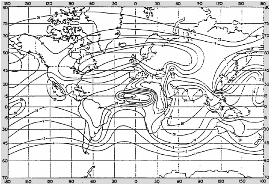
时间梯度百分比 \leq -100 (N- units/km) : 二月
