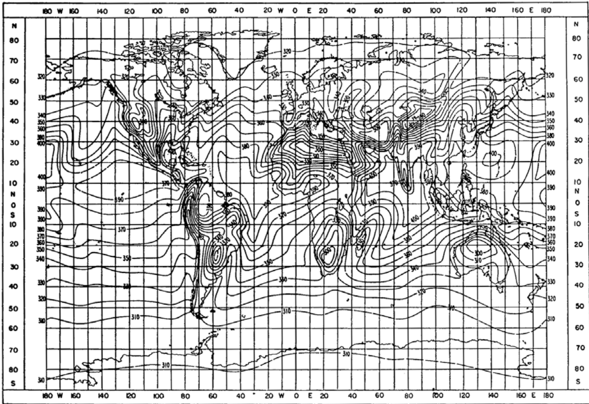
图2 M月平均值：八月
