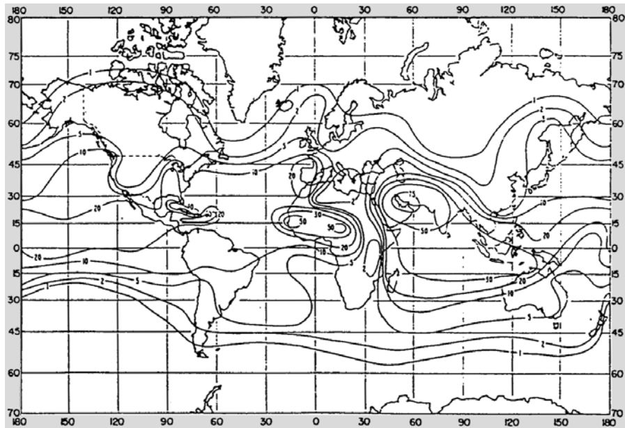
时间梯度百分比 \leq -100 (N- units/km) : 五月
