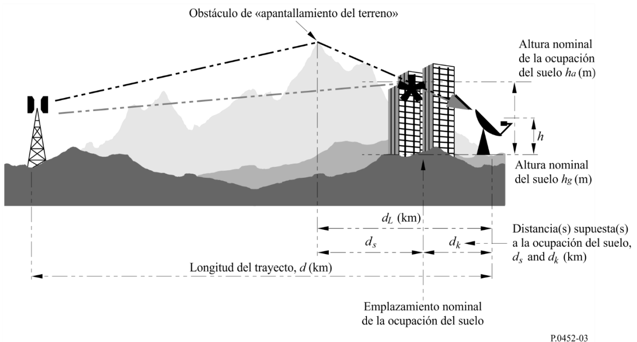
FIGURA 3 Método de aplicación de la corrección altura-ganancia, A_{hr} o A_{hr}
