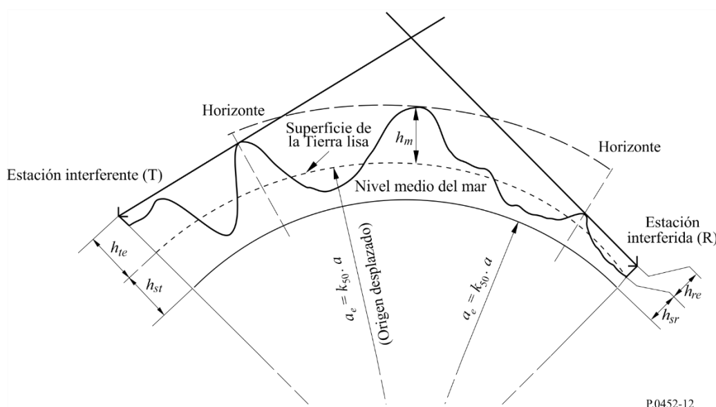
Ejemplo de superficie de la Tierra lisa y del parámetro de rugosidad del terreno
