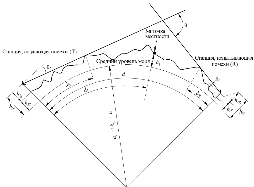
РИСУНОК 11 Пример профиля (загоризонтной) трассы
