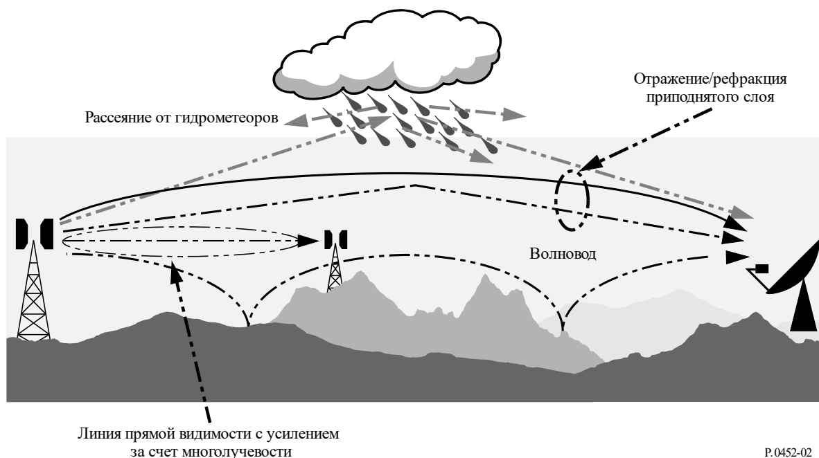
РИСУНОК 2 Аномальные (краткосрочные) механизмы распространения помех
