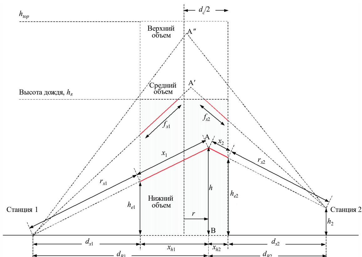
РИСУНОК 9 Объемы интегрирования в пределах очага дождя
