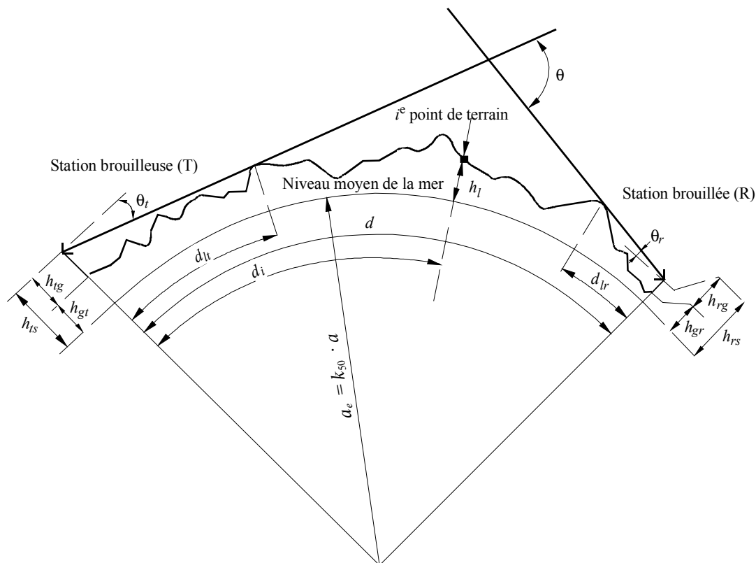
Exemple d'un profil de trajet (transhorizon)
