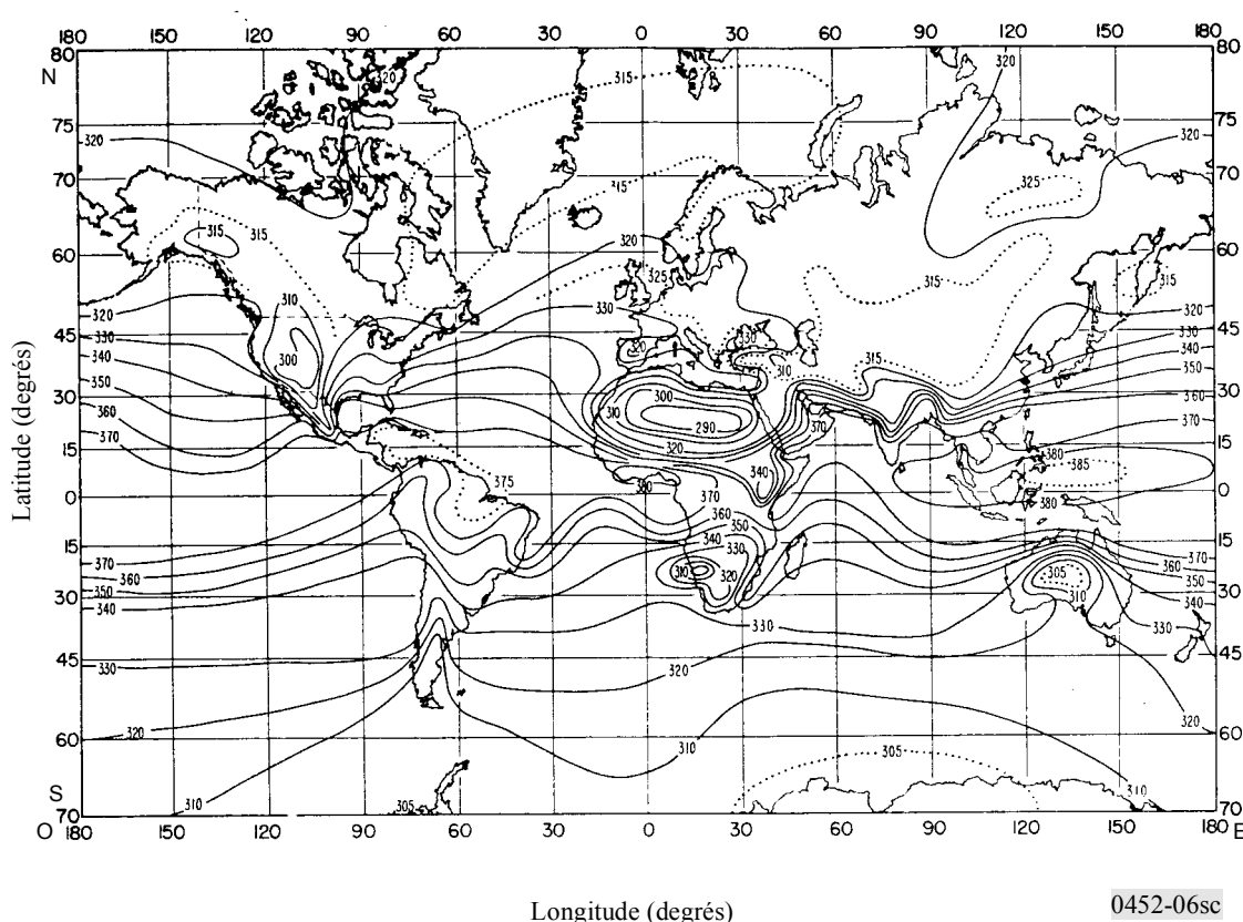
FIGURE 6 Coïndice au niveau de la mer, N_0
