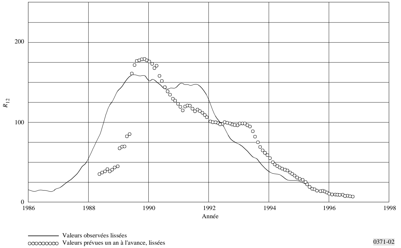
FIGURE 2 Exemple de nombres de taches solaires, R_{12} , prévus et observés (cycle 22)
